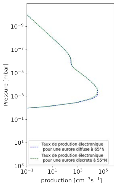
Figure V.18: Taux de production électronique modélisés pour les régions des aurores discrètes, à 55°N, et des aurores diffuses à 65°N. Ces taux de production sont calculés en utilisant le modèle d’atmosphère neutre initialement introduit dans la modélisation Trans-Planet.
