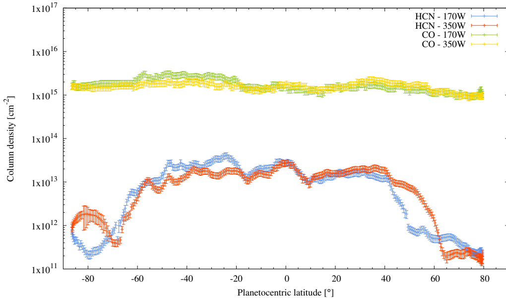
Figure V.7: Densité de colonne de HCN et CO en cm^{-2} aux longitudes des deux limbes observés en fonction de la latitude planétocentrique.
