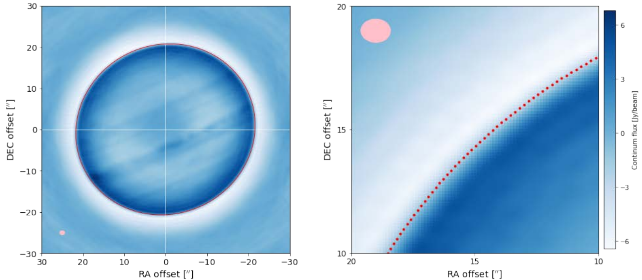
Figure III.1: À gauche est représenté le continuum de la bande spectrale HCN. En rouge est représentée l'ellipse correspondant à la position géométrique du limbe apparent de Jupiter. À droite, un agrandissement d'une région du limbe au côté ouest du disque planétaire apparent. Les points rouges au limbe correspondent aux pointages calculés et où les raies spectrales seront extraites du cube de données.
