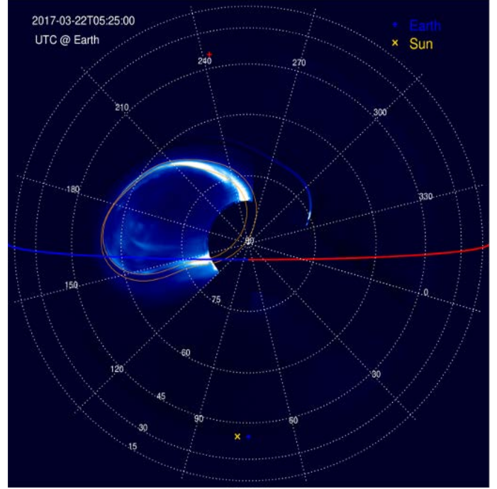
(b) HCN
