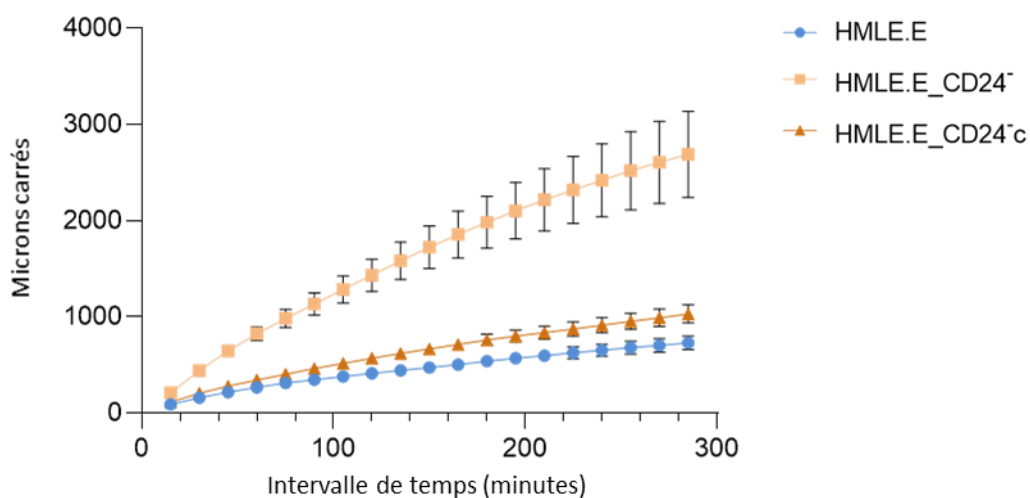
Figure 27 - Déplacement moyen quadratique des cellules HMLE.E, HMLE.E CD24 - , HMLE.E CD24 c
