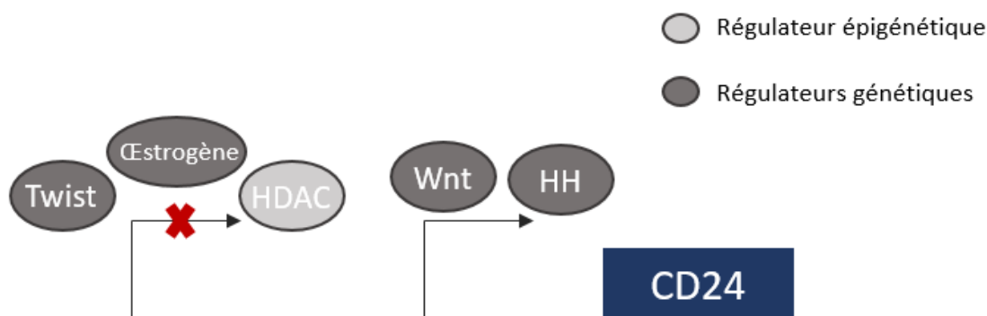
Figure 15 - Régulation transcriptionnelle de CD24
