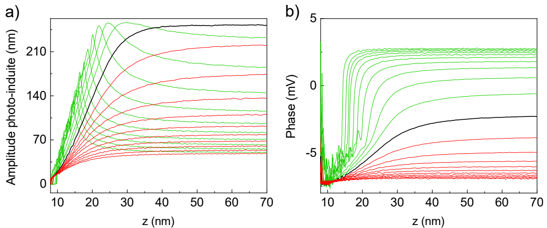
FIGURE 3.10 – Dépendance de l'amplitude photo-induite vis à vis de la fréquence de modulation f_{mod} . Évolution spatiale de l'amplitude photo-induite (a) et de la phase (b) avec \Delta f variant de +50 Hz jusqu'à -50 Hz. La couleur des courbes dépend de la modulation initiale : sub-résonance en vert, supra-résonance en rouge et f_{mod} = f_0 en noir. Le levier recouvert de nanoparticules d'or a été utilisé ici.
