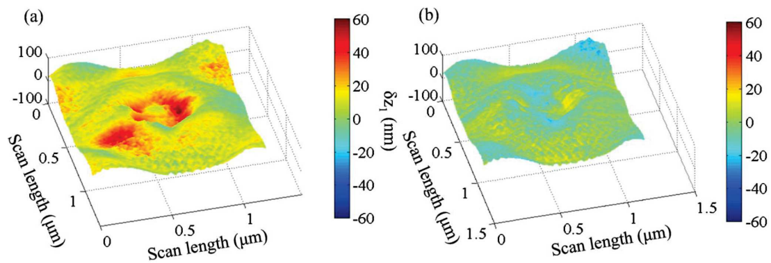
FIGURE 1.14 – (a) Différence \delta z_1 = z_{ON} - z_{OFF} entre les signaux de topographie d'une surface illuminée et d'une surface non illuminée. (b) Différence \delta z_2 = z_{OFF1} - z_{OFF2} entre deux signaux de topographie sans illumination, permettant de détecter les erreurs dues à la mesure [66].
