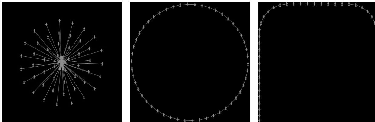
FIGURE 5.7 – Visualisation des structures de réseaux en étoile, cycle et ligne
