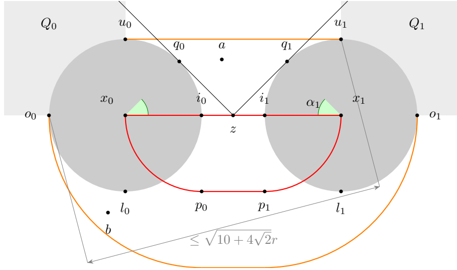
FIGURE 2.30 – La figure illustre les notations utilisées dans la preuve du lemme 2.3.13. La preuve consiste à montrer que l'un des deux chemins rouges joignant x_0 et x_1 est inclus dans A \ominus \bar{B}(0, r) .
