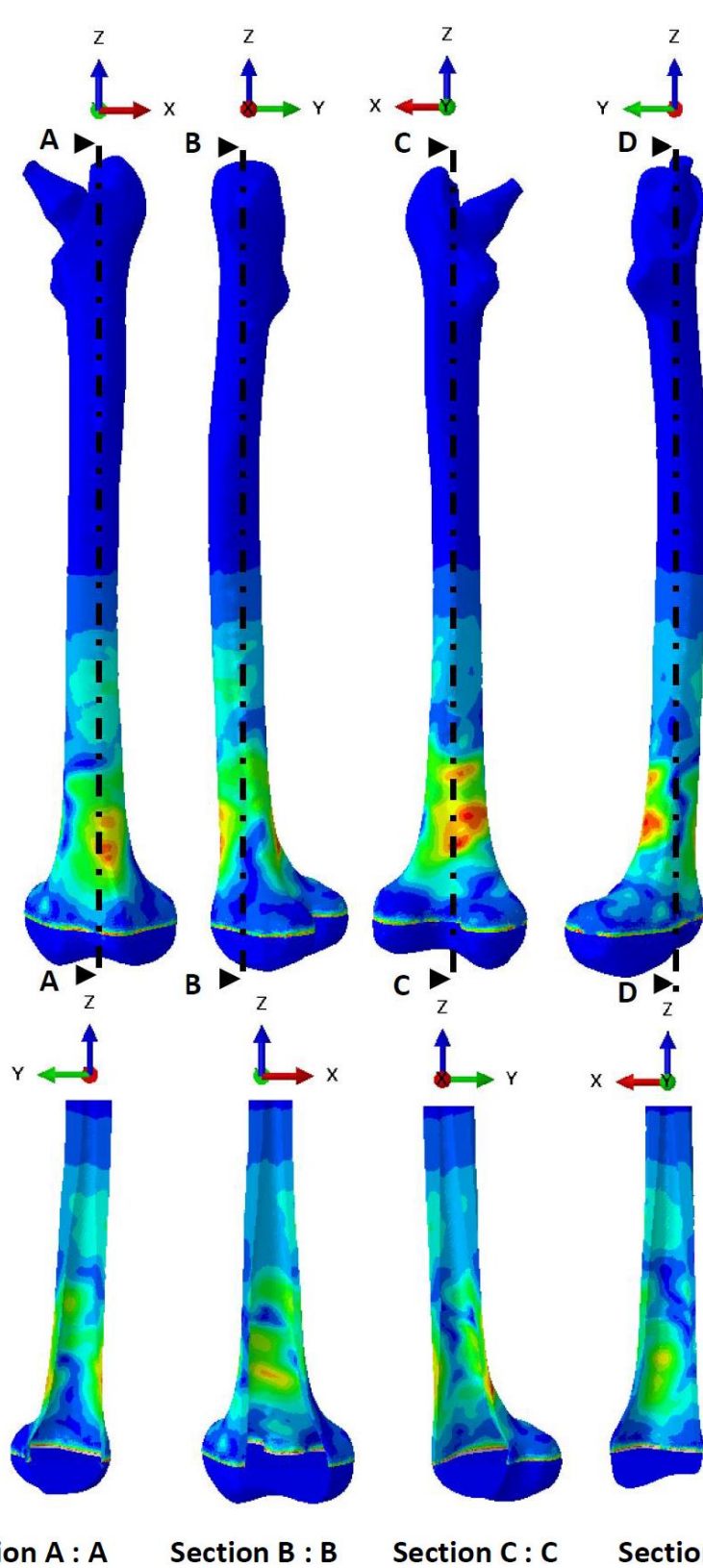
Figure 15 : Distribution de la contrainte de Von Mises équivalente [MPa] à l'extérieur et à l'intérieur de la couche corticale d'un fémur avec une prothèse de genou repliée (uniquement le composant du genou) lors d'une simulation d'impact frontal au moment de l'impact.
