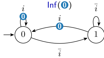
(a) Automate de Büchi associé à \text{GF}(i)
