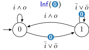
(a) Automate de Büchi associé à \mathbf{GF}((i \wedge \bar{o}) \vee \bar{i})
