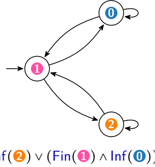
(b) Automate de parité maximale paire totalement colorié
