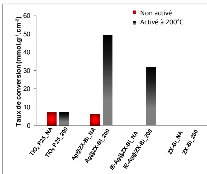
Figure V-5 : Taux de conversion du méthanol (en mmol par gramme de catalyseur par cm 2 de surface irradiée) après 720 min (12h) de réaction. Conditions de réaction : [MeOH]=10350 ppm (1%) dans 20% O 2 /Ar; m_{\text{catalyseur}} = 20 mg; Lampe Xe avec un filtre ( \lambda > 390\text{nm} ) ; irradiance = 71 mW/cm 2 ; Débit total = 25 cm 3 /min. Catalyseurs activés à 200 °C sous Ar pendant 30 min dans l'obscurité suivi de 30 min d'irradiation visible.
