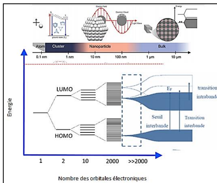
Figure I-1 : Schéma représentatif de la structure électronique caractéristique des métaux nobles en passant de l'état atomique à l'état massif.
