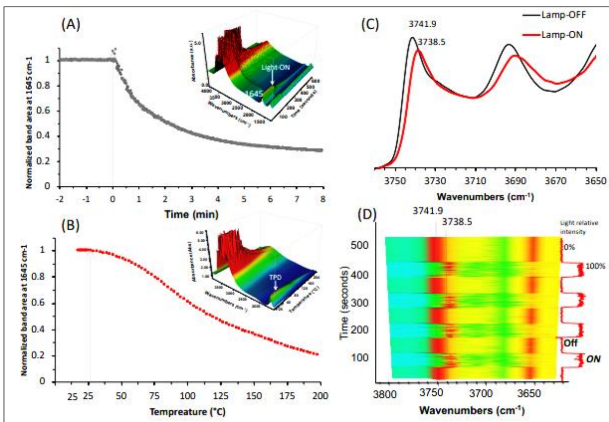
Figure IV-15 : Evolution de la zone de bande IR (centrée à 1645 cm -1 ) de l'eau adsorbée sur les échantillons Ag@ZX-Bi-3 en fonction (A) du temps d'irradiation en lumière visible à 25°C, et (B) de la température dans l'obscurité. Insert : cartographie 3D des spectres originaux correspondants. La flèche correspond à l'allumage de la lumière (t=0s) et au point de départ chauffage (taux = 1,75°C/min), respectivement. Conditions expérimentales : débit d'Ar (25 cm 3 /min) ; m cat =20 mg (pastille de 2 cm 2 de diamètre et 65 μm d'épaisseur ; source lumineuse utilisée dans (A) lampe Xe avec filtre UV coupé (λ>390 nm) et irradiane ≈ 150 mW/cm 2 . (C) Spectres IR de l'échantillon Ag@ZX-Bi dans la région de vibration du SiOH dans l'obscurité (noir ; lampe éteinte) et sous irradiation visible (rouge; lampe allumée). Echantillon activé à 28°C sous lumière visible pendant 30 min. (D) Cartographie 2D de la variation d'intensité de la bande dans la région 3800-3650 cm -1 à différents cycles de lampe éteinte/lampe allumée (le rouge et le bleu-vert correspondent respectivement à l'intensité supérieure et inférieure). (Intensités relatives lumineuses (0% ou 100%) : position basse : volet fermé ; position haute : volet ouvert). L'axe de l'échelle verticale correspond au temps des expériences. Remarque : (C) et (D) ont été mesurés sur le même échantillon et dans les mêmes conditions que celles utilisées en (A).
