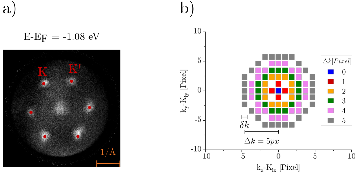
FIGURE 5.8 – a) Coupe isoénergétique à travers la zone de Brillouin pour une MC-WSe_2 sur hBN à E - E_F = 1.08 eV, c'est-à-dire peu dessous le haut de la bande de valence. A cette énergie, des domaines de haute photointensité apparaissent. Leurs centres marquent les positions des points K et K' . b) Positions de spectres « équivalents » dans l'espace réciproque autour d'un point de haute symétrie K/K' ou \Gamma qui est placé au centre. Les valeurs du \mathbf{k} sont discrétisées en pixels. Grâce à l'isotropie autour d'un point de haute symétrie, les spectres qui remplissent \left| |\mathbf{k} - \mathbf{K}_i| - \Delta k \right| \leq \delta k/2 pour le même \Delta k devraient avoir la même forme (ils sont « équivalents »). Ici, \delta k est la largeur réciproque d'un pixel. Cette condition est valable pour \Delta k \leq \overline{\Gamma K} [78].
