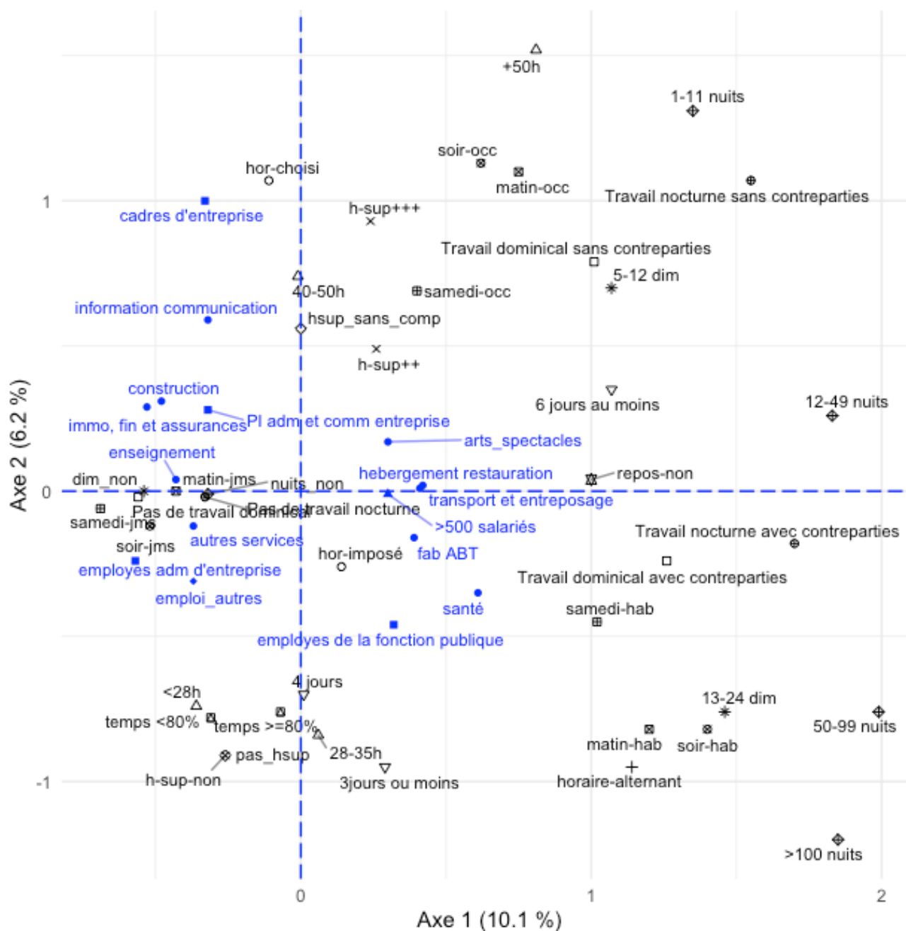
Figure 4 – Représentation graphique des variables actives et supplémentaires sur les axes 1 et 2
