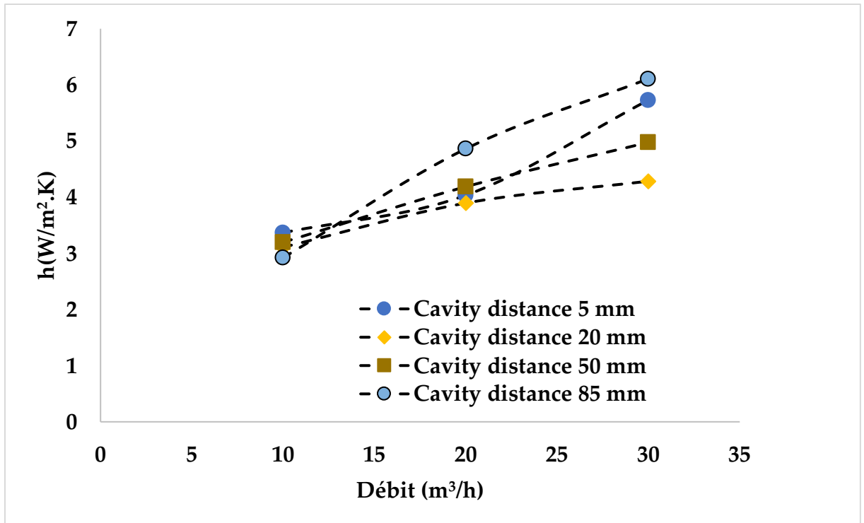
Figure 3.23 Le coefficient convectif dans la lame d'air
