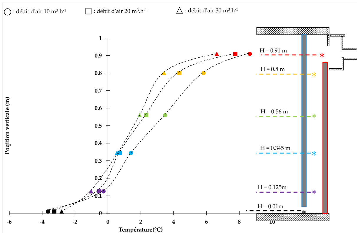
Figure 3.11 Évolution de la température à l'intérieur de la chambre à air pour une distance entre les parois de 85 mm pour les débit d'air (10 m 3 .h -1 , 20 m 3 .h -1 et 30 m 3 .h -1 )
