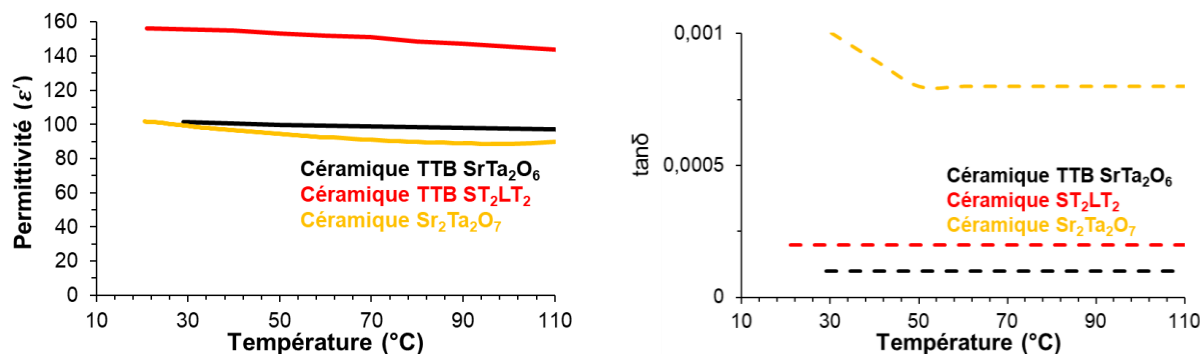
Figure 3.9 : Evolution (a) de la permittivité et (b) des pertes à 10 kHz en fonction de la température de céramiques TTB SrTa_2O_6 et ST_2LT_2 , frittées à 1595°C, et de la céramique perovskite STLTO de composition x=0 .
