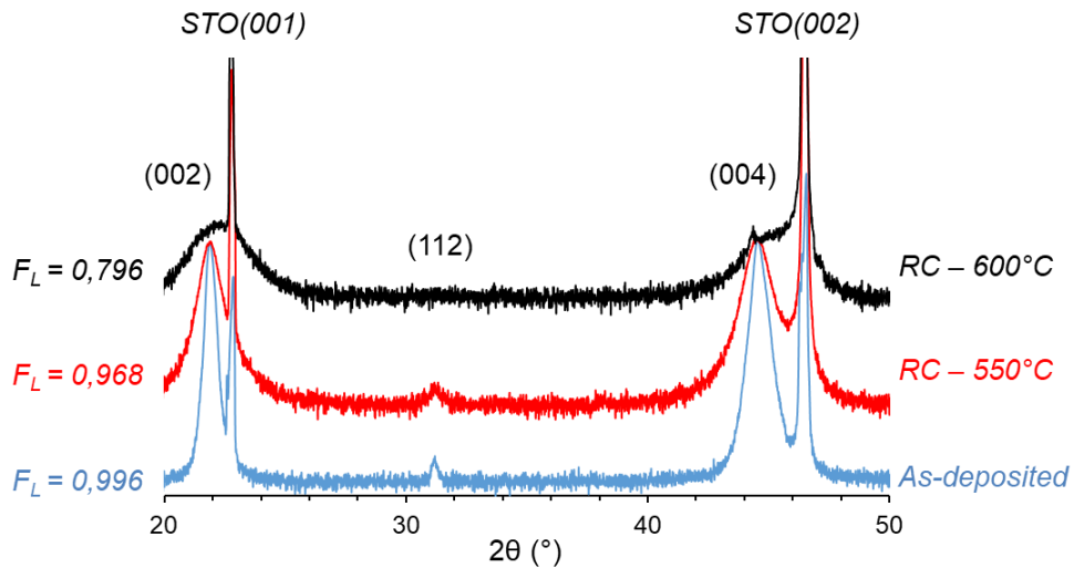
Figure 4.3 : Diagrammes de diffraction des rayons X des couches minces FSTLTON, déposées par pulvérisation cathodique sur Nb-SrTiO 3 à T_S = 800^\circ\text{C} , avant (« as-deposited ») et après recuit ex-situ (RC) pendant 4 heures à 600^\circ\text{C} et 550^\circ\text{C} .
