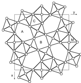
Figure 1.15: (a) Projection schématique le long de l'axe \vec{c} de la maille TTB A_2BC_2M_5X_{15} et localisation des sites cationiques A, B et C et (b) nature des ions pouvant occuper les sites cristallographiques [73].
