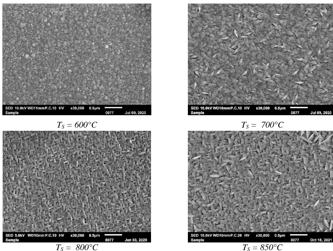
Figure 4.19 : Morphologies de surface vues par MEB des couches minces FSTLTO déposées par pulvérisation cathodique sur MgO sous argon pur en variant la température de dépôt T_S .
