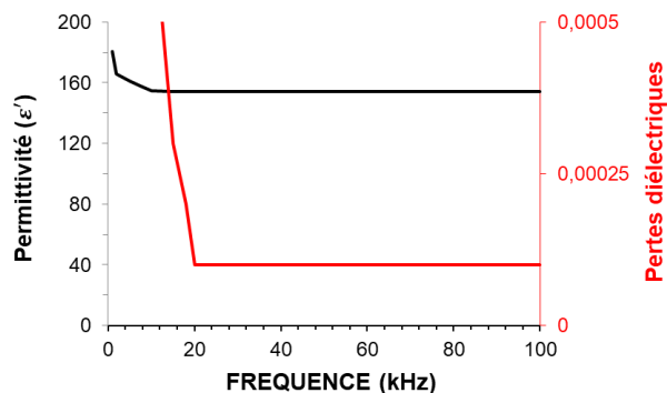
Figure 3.8 : Evolution de la permittivité et des pertes diélectriques de la céramique \text{ST}_2\text{LT}_2 en fonction de la fréquence entre 1 et 100 kHz.
