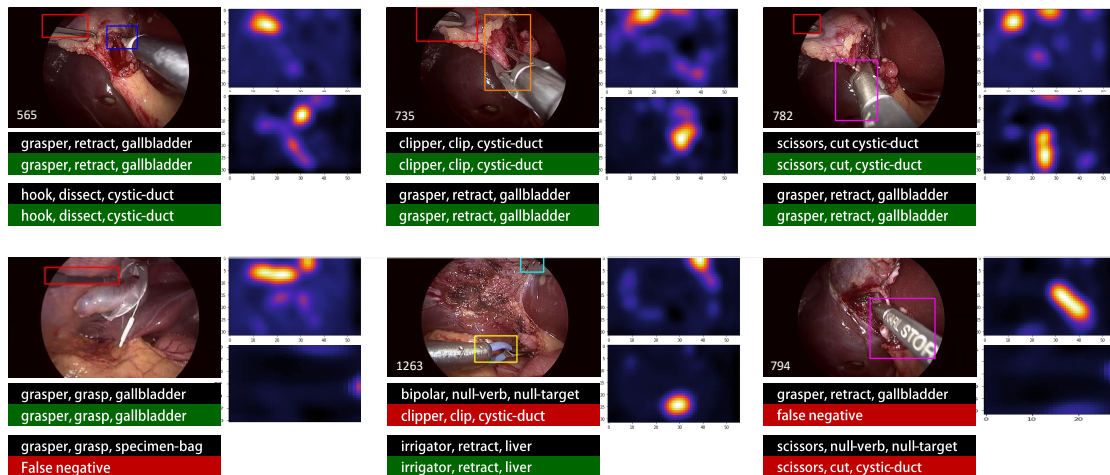
Figure B.10 – Résultats qualitatifs du modèle RDV montrant les prédictions de triplet et les cartes thermiques pour la détection de triplet. Les cadres de délimitation de localisation sont obtenus à partir du module WSL du modèle RDV proposé. Les triplets prédits et vérité terrain sont affichés sous chaque image : noir = vérité terrain, vert = prédiction correcte, rouge = prédiction incorrecte. Un triplet manqué est marqué comme faux négatif et une fausse détection est marquée comme faux positif.
