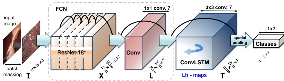
Figure B.4 – L’architecture du Traqueur ConvLSTM proposé.
