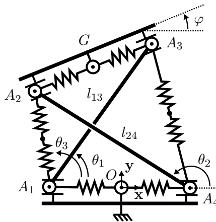
FIGURE 2.2 – Croix de Snelson de référence utilisée pour construire les mécanismes.
