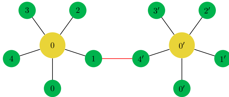
FIGURE 3.12 – Les configurations en étoile sont révélatrices de la présence des noyaux. Les segments de Bord sont représentés en vert et ceux de Centre sont en jaune. Les arêtes en noir sont les fusions prioritaires. La fusion rouge est une liaison \text{Bord} \Leftrightarrow \text{Bord} et doit être réalisée plus tard sous peine de créer des motifs absurdes.
