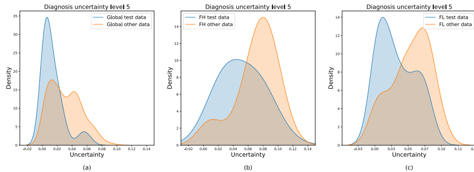
FIGURE 2.15 – Comparaison des distributions de l’indice de confiance entre les données de test familiaires, HF/LF , et d’autres données moins familiaires non-HF/LF . Les distributions sont données pour le diagnostic global (a) et le diagnostic spécifique à chaque classe (b et c). Nous séparons les distributions de test (courbes bleues) et les distributions non familiaires (courbes oranges) sur chaque graphe. Les lames non-HF/LF sont diagnostiquées avec une plus grande dispersion (indice de confiance plus faible) que celle observée dans les données HF/LF .
