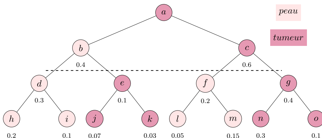
FIGURE 3.5 – Arbre de subsomption. Chaque nœud est un concept identifié par une lettre. Les couleurs indiquent la présence d'une classe majoritaire, « peau » ou « tumeur » pour reprendre l'exemple de la Figure 3.2 et de la Figure 3.3. Les concepts situés sous la ligne en pointillés sont purs , c'est-à-dire que leur définition \mathbf{I}(\text{concept}) ne contient que des éléments de la classe dans laquelle ils sont colorés. Sous chaque concept se trouve la fraction de patches du concept-racine a qui lui est rattachée.
