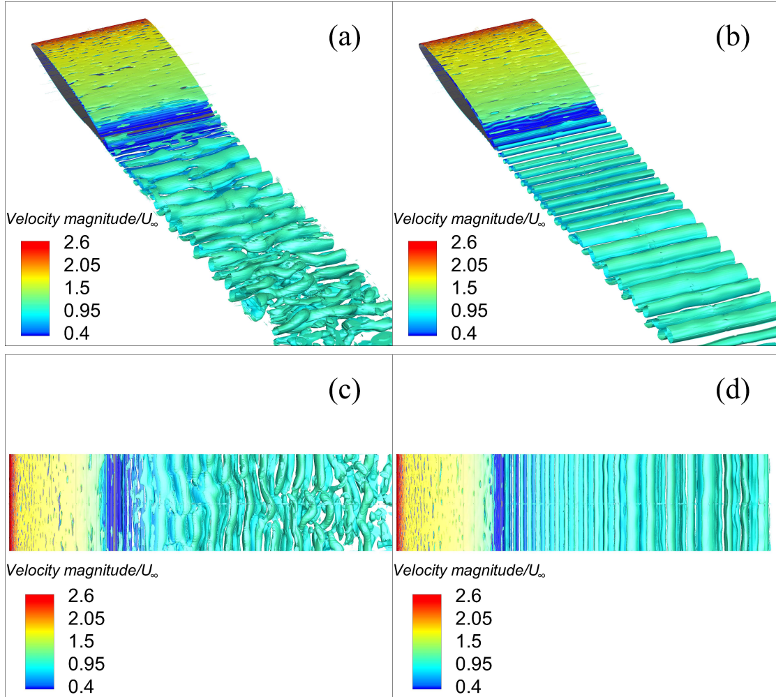
FIGURE 2: iso-surfaces du Q-critère ( Q=1500 ) coloré avec le champs de la vitesse non-dimensionnelle. (a) and (c) cas statique (pas de vibration), (b) and (d) cas morphing (avec vibration).
