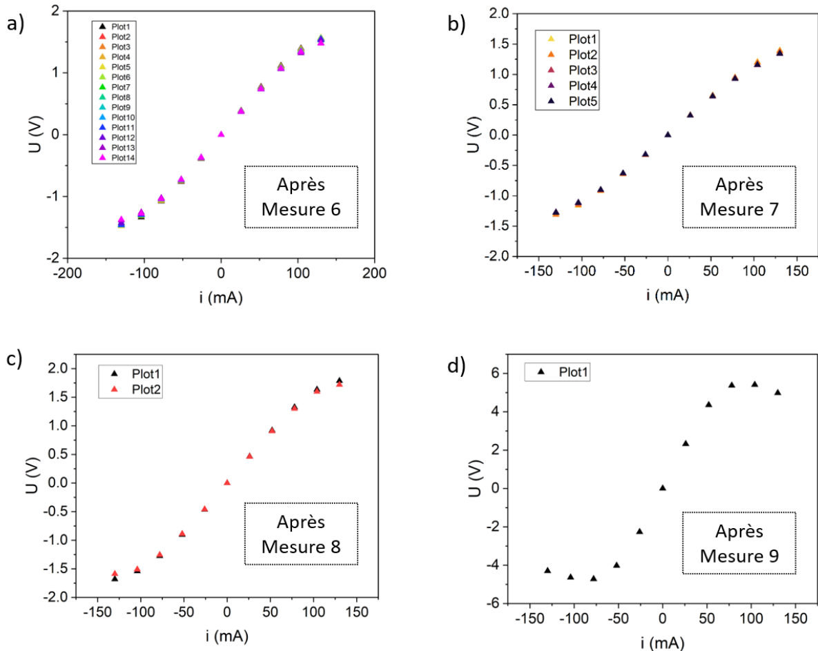
FIGURE III.19 – Courbes U = f(i) sur l'échantillon \text{Rb}_{0,2}\text{Ba}_{0,4}\text{Cr}_5\text{Se}_8 après mesures de propriétés avec i_{\text{max}} = 130 mA. a) Succession de quatorze courbes enregistrées d'affilée après la mesure 6, b) Cinq courbes après la mesure 7, c) Deux courbes après la mesure 8, d) Courbe après la mesure 9.
