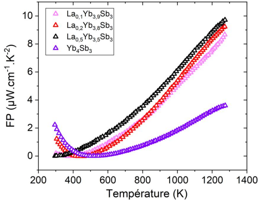
FIGURE V.4 – Facteur de puissance du composé binaire Yb_4Sb_3 et des composés dopés La_xYb_{4-x}Sb_3 ( x = 0,1 ; 0,2 ; 0,5 ). Tiré de [208].
