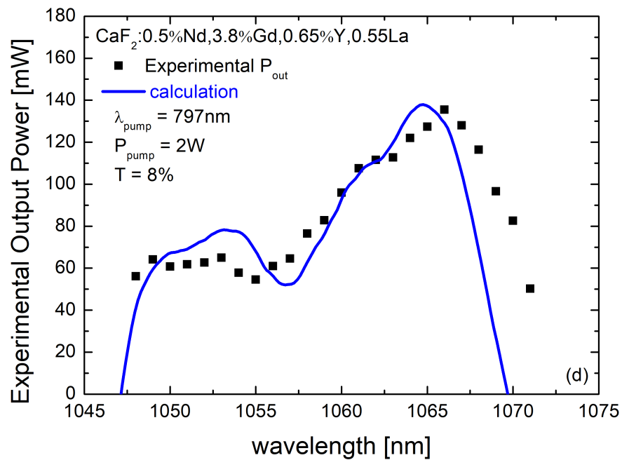
FIGURE 11: Courbes d'accord et reconstruction d'un \text{CaF}_2 : 0.5%Nd co-dopé avec 2.5%Gd,2.5%Y (a), 4%Gd,1%Y (b), 3%Gd,1.4%Ce,0.6%Y (c) and 3.8%Gd,0.55%La,0.65%Y (d).
