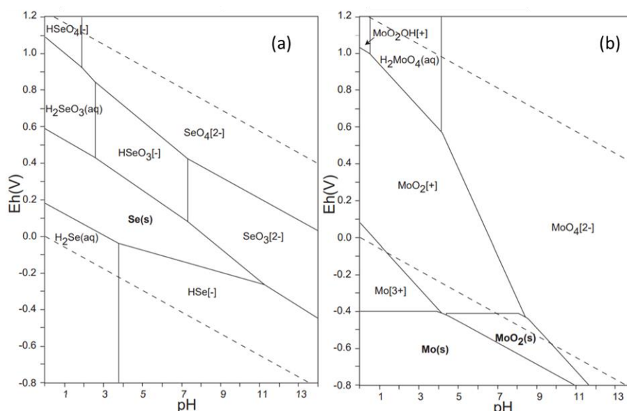
Figure 1-7 : Diagrammes de prédominance Eh-pH du Se (a) et du Mo (b) compilés à partir de la base de données thermodynamiques HATCHES (Taneko, 2005)
