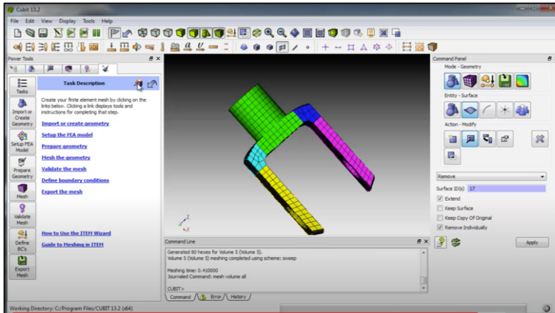
Figure 2.27 – Exemple du logiciel Cubit avec lequel un utilisateur découpe son modèle géométrique en morceaux pour lesquels un maillage par balayage est applicable.
