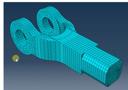
Figure 2.28 – Exemple du logiciel Abaqus avec lequel un utilisateur découpe son modèle géométrique en blocs simples qui seront ensuite discrétisés par des grilles.
