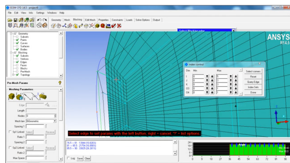
Figure 2.29 – Les logiciels MGX (à gauche) et ICEM-CFD Hexa (à droite) sont basés sur la construction d'une structure de blocs qui s'appuie sur un domaine géométrique sans le découper ou le modifier.
