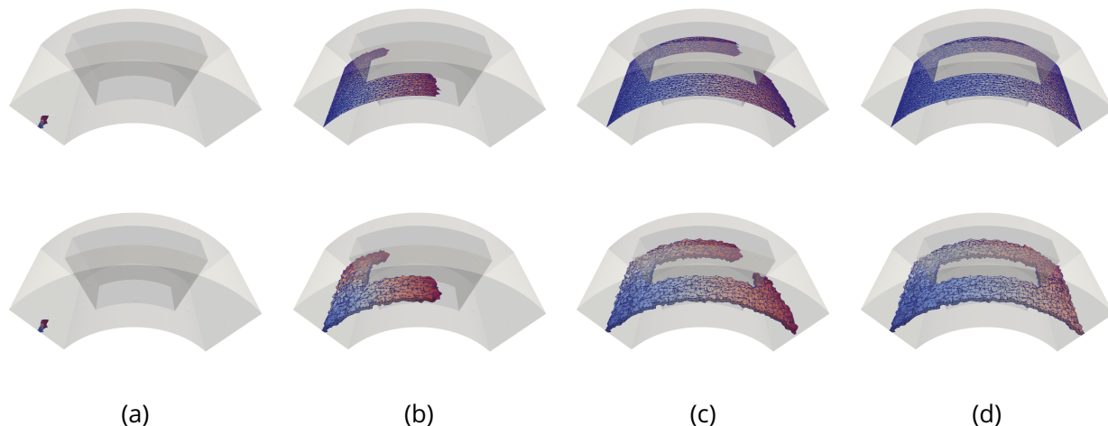
Figure 3.8 – Illustration de la création de feuillet dans un champ régulier : Sur la ligne du haut, une représentation surfacique de l'avancée du feuillet dual. En (a), on commence à partir d'un seul tétraèdre et ensuite on avance en (b) et (c) dans le domaine en suivant le champ d'orientation jusqu'à atteindre le bord du domaine dans toutes les directions de propagation en (d). La couleur d'un élément (un morceau de la surface ou un tétraèdre) est corrélée avec l'indice de la vague de propagation.
