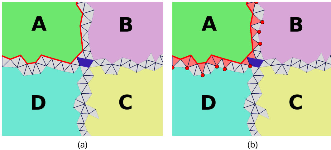
Figure 3.39 – Ici nous cherchons les régions duales voisines de la région duale A . En (a) nous atteignons le bord (en rouge) de la région duale en contact avec les feuillettes duales et en (b) nous traversons ces feuillettes duales pour entrer en contact avec les régions duales voisines.
