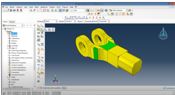
Figure 2.28 – Exemple du logiciel Abaqus avec lequel un utilisateur découpe son modèle géométrique en blocs simples qui seront ensuite discrétisés par des grilles.
