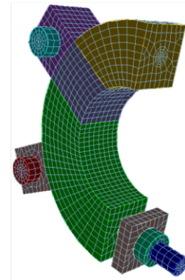
Figure 2.27 – Exemple du logiciel Cubit avec lequel un utilisateur découpe son modèle géométrique en morceaux pour lesquels un maillage par balayage est applicable.
