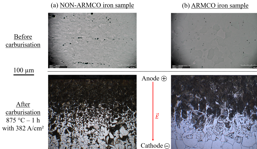
Figure 1: Micrographies optiques des microstructures avant et après 1 h de carburation à 875 °C avec 382 A cm -1 . (a) L'échantillon de fer NON-ARMCO à gauche, comparé à (b) l'échantillon de fer ARMCO à droite.
