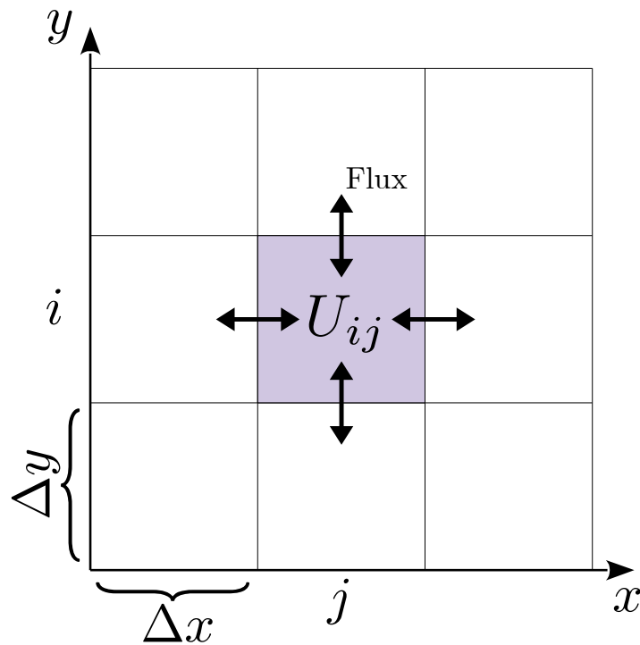
Figure 6.1 – Illustration de la méthode de discrétisation pour les volumes finis, ici en 2D sur une grille uniforme.
