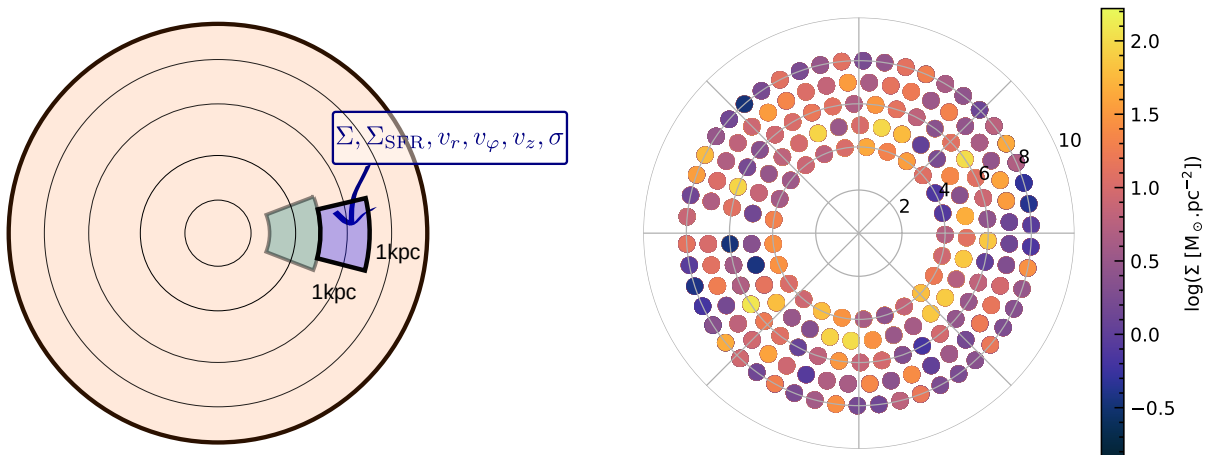
Figure 11.2 – Schéma d'un secteur de 1 \text{ kpc}^3 dans le disque galactique (gauche), et position des différents secteurs de la zone d'analyse (droite). Les chiffres indiquent le rayon en kiloparsec, et la couleur de chaque secteur correspond à sa densité de colonne moyenne dans la simulation F20.
