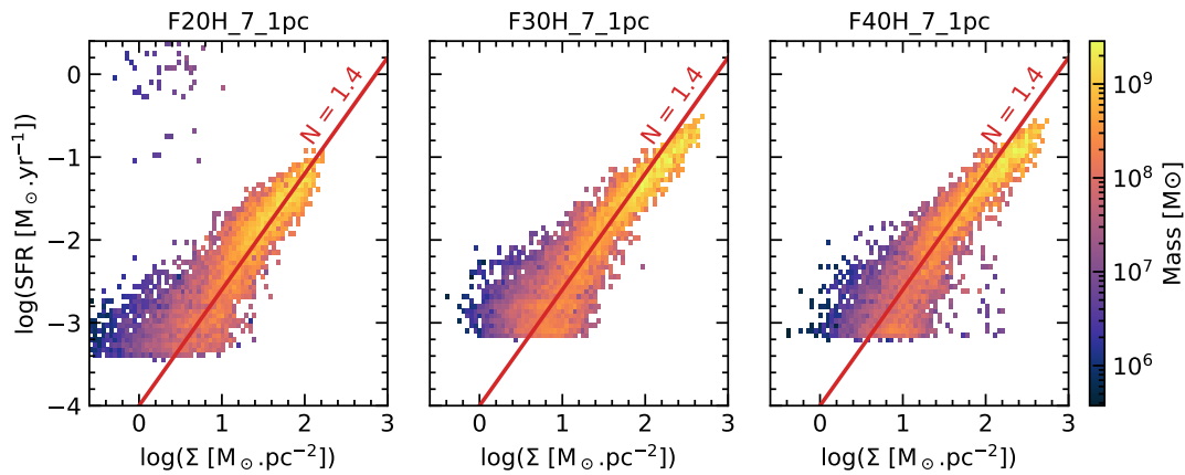
Figure 11.4 – Loi de formation d'étoile dans des régions de 1 \text{ kpc}^3 . Le SFR mesuré peut être assimilé à une densité de surface de SFR ( \Sigma_{\text{SFR}} en M_{\odot} \cdot \text{yr}^{-1} \cdot \text{kpc}^{-2} et ainsi être comparé à la relation de Schmidt-Kennicutt. Cette figure compile les valeurs du SFR entre 100 et 300 Myr.
