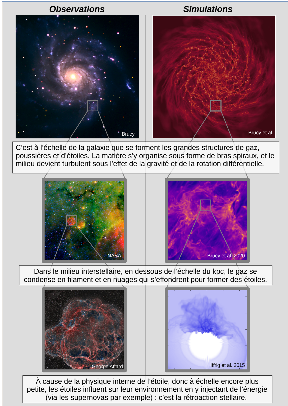
Figure 1.5 – Les différentes échelles étudiées dans cette thèse. Les trois lignes correspondent à des illustrations d'une galaxie à trois échelles différentes, mais il ne s'agit pas de réels agrandissements.
