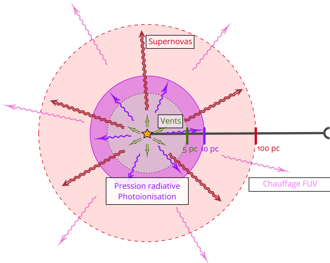
Figure 4.1 – Les différents modes de rétroactions stellaires et leurs échelles typiques. Les supernovas marquent la fin de la vie d'une étoile et ne sont pas simultanées aux autres formes de rétroactions. Les rétroactions de plusieurs étoiles massives proches peuvent se combiner, mais pas nécessairement linéairement.
