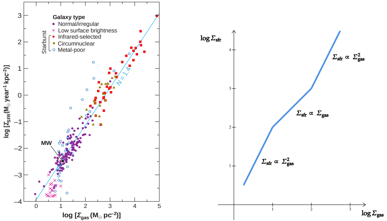
(a) Relation entre la densité de colonne de gaz totale (atomique et moléculaire) et la densité de colonne de SFR (Kennicutt & Evans, 2012).
