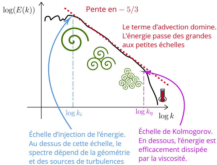
Figure 4.4 – Exemple de spectre d'énergie illustrant une cascade turbulente (cas incompressible homogène).
