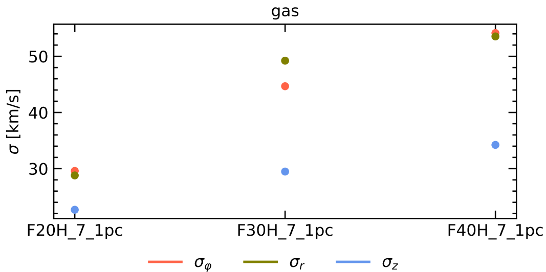
Figure 11.5 – Dispersion de vitesse azimutale, radiale et verticale moyennée dans toutes la zone d'analyse.
