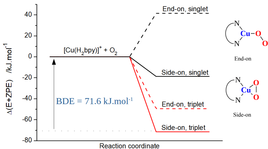
Figure 5: Diagramme de stabilité des différents adduits [Cu(H_2bpy)(O_2)]^+ en fonction de leur mode de coordination et de leur état de spin.
