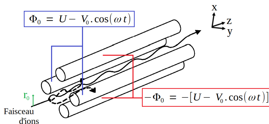
Figure 10: Schéma de l'analyseur quadripolaire (les flèches en pointillés représentent des trajectoires instables)
