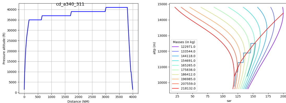
(a) Exemple de profil de vol calculé avec le module de mission pas-à-pas. (b) Évolution de la SAR au cours du vol représenté pour les altitudes de croisière
