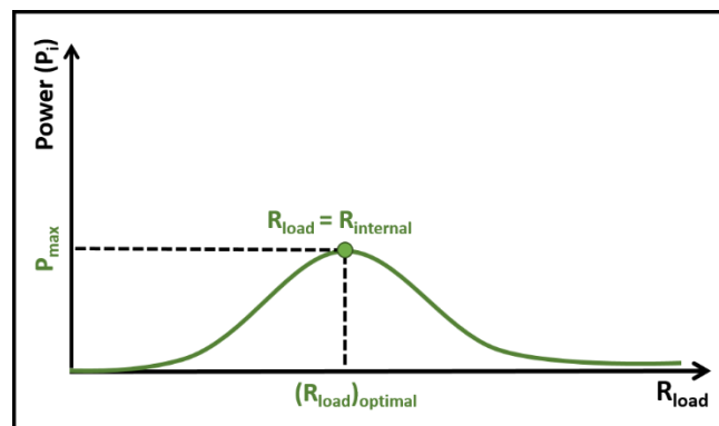
Figure 3. Représentation théorique de la courbe de puissance en fonction de R_{load} . Le maximum de la courbe est obtenu lorsque la R_{load} est égale à la résistance interne du système mesuré.
