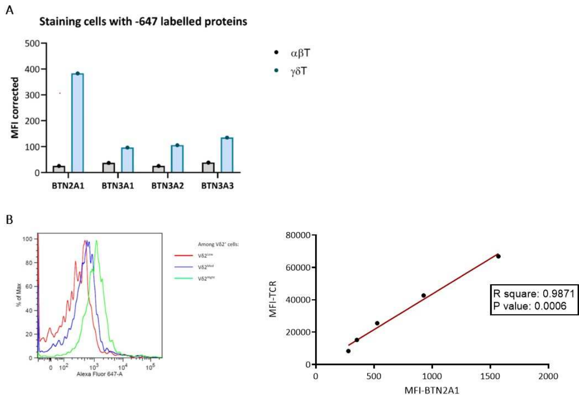
Figure 22 Un monomère de BTN2A1 est suffisant pour fixer des LT V\gamma 9V\delta 2 de façon TCR-dépendante. Les monomères de protéines synthétisées pour l’ancrage dans les SLB sont utilisées comme des anticorps de marquage. (A) Comparaison du marquage obtenu pour chaque BTN sur des LT V\gamma 9V\delta 2 ou des LT \alpha\beta et (B) corrélation de l’intensité de marquage obtenu avec BTN2A1 sur des LT V\gamma 9V\delta 2 .
