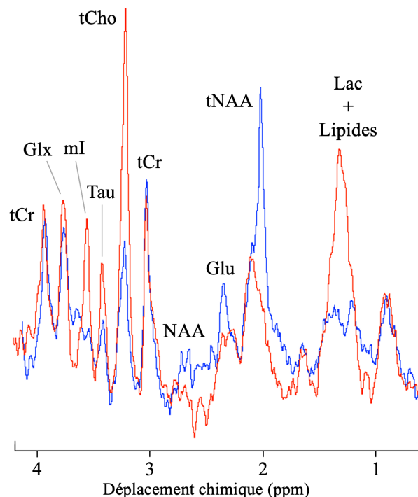
Figure 4.17. Superposition du spectre RMN ^1\text{H} in vivo typique du tissu cérébral sain (en bleu) et du spectre RMN ^1\text{H} in vivo typique du tissu cérébral tumoral (en rouge). Les deux spectres RMN ont été acquis avec les micro-antennes RMN implantables (volume de détection = 1 \mu\text{L} ). Signaux : tCho : choline totale, tCr : créatine totale, tNAA : NAA total, Tau : taurine, mI : myo-inositol, Glx : glutamine + glutamate, Lac : lactate.
