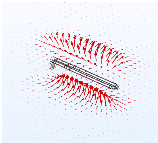
Figure 3.9. Champ magnétique \vec{B}_1 généré par la boucle résonante de la micro-antenne « loop » ayant une largeur de 450 \mu\text{m} . Les flèches rouges sont proportionnelles à l'amplitude de \vec{B}_1 .
