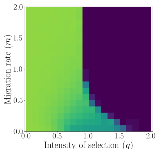
(d) IBS outcomes - 10 loci.
