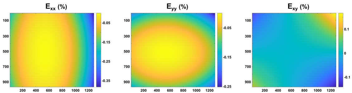
FIGURE 2.6 – Erreur sur les déformations E_{xx} (gauche), E_{yy} (milieu) et E_{xy} (droite) liée à la distorsion de la caméra en fonction de la position sur le champ de vue.
