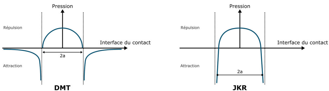
FIGURE 1.9 – Schématisation des distributions de pression modélisées par les théories de DMT (gauche) et de JKR (droite).
