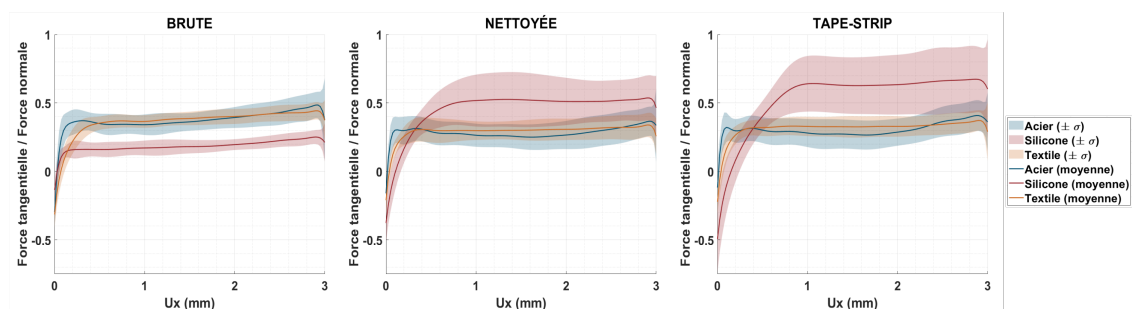
FIGURE 2.12 – Évolution du ratio de la force tangentielle sur la force normale (moyenne et écart-type ( \sigma )) lors du dernier cycle de frottement pour chaque condition de contact. À gauche pour les échantillons bruts, au milieu pour les échantillons dont la surface a été nettoyée, à droite pour les échantillons nettoyés et endommagés par tape-stripping.
