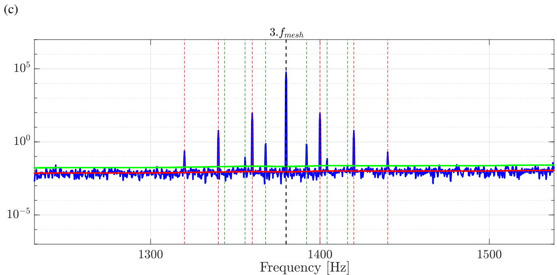
FIGURE 3.14: Estimation spectrale du bruit VAI à l'aide du périodogramme moyenné ( M=5 ) : VAI estimée superposée à la VAI réelle (a), périodogramme de l'enveloppe du signal filtré en noir avec sa moyenne glissante à 200 échantillons en bleu (b), périodogramme de la VAI (c) : la ligne bleue indique le périodogramme de la VAI, le périodogramme moyen à 200 échantillons en noir, la ligne rouge est le bruit VAI estimé, la ligne jaune est le seuil de bruit VAI avec \alpha = 1\%
