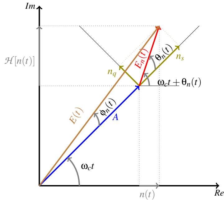
FIGURE 3.5: Représentation complexe d'un signal harmonique bruité
