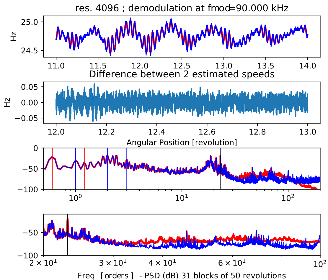
FIGURE 4.10: Comparaison entre la méthode ET (bleu) et la technique de démodulation haute fréquence (rouge). La courbe du haut montre la vitesse instantanée de l'arbre estimée par les deux méthodes. La différence est tracée en dessous. Les courbes du bas montrent les spectres correspondants. Les lignes verticales correspondent aux fréquences d'entrée (en bleu) et de sortie (en rouge) de l'arbre et à leurs harmoniques respectives.
