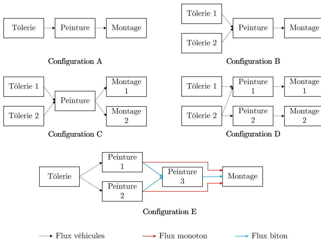
Figure 1.4 – Configurations d'usines d'assemblage automobile
