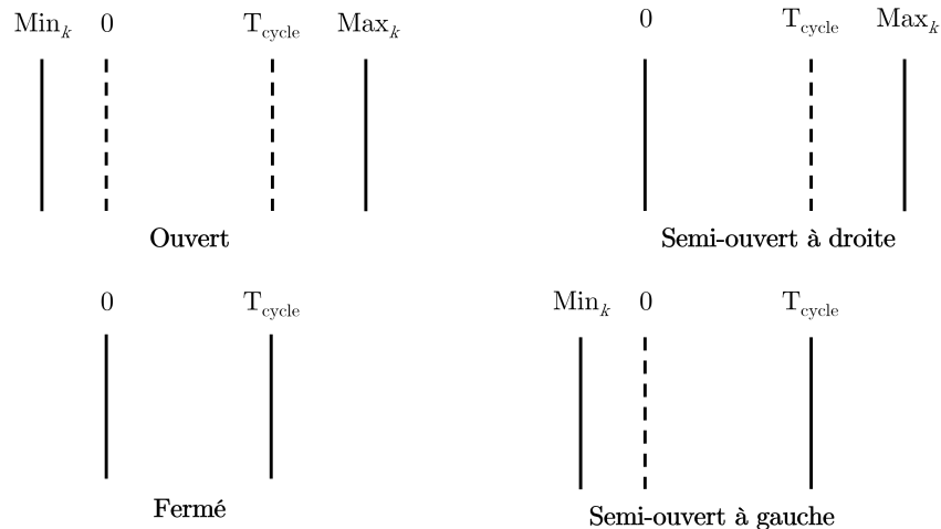
Figure 2.3 – Quatre configurations de postes de travail d’après Cevikcan & Durmusoglu (2011)
