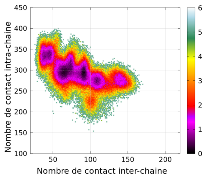
FIGURE 2.14 – Exemple typique de carte de couleur du nombre de contacts intra-chaine en fonction du nombre de contact inter-chainnes pour les dimères du WT.
