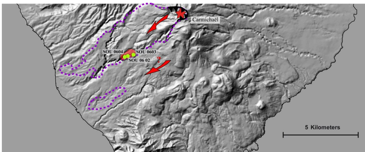
Figure VI.38 : Carte des différents affleurements étudiés de la phase PMD 10. En pointillé violet est représentée l'extension déduite de l'avalanche de débris AD 10.
