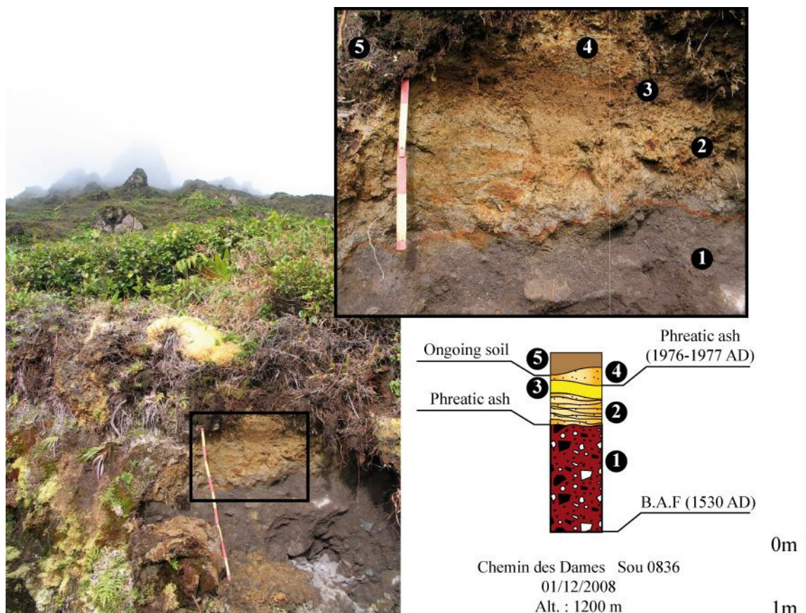
Figure V.6 : Description des niveaux de retombées de cendres des éruptions phréatiques historiques observées sur l'affleurement du Chemin des Dames (SOU 0836).
