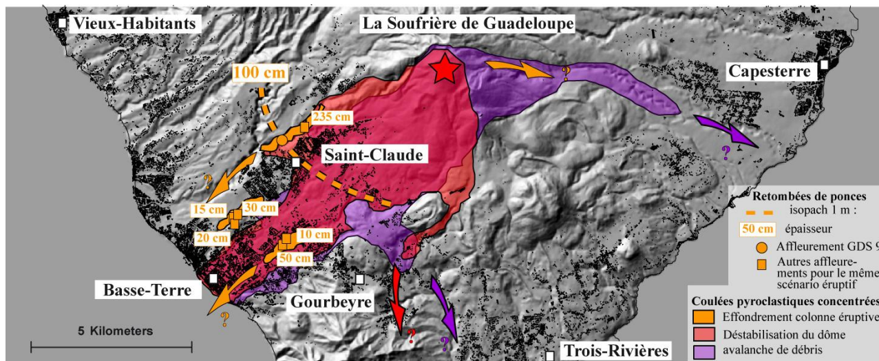
Figure VII.11 : Cartographie interprétée des zones impactées par les dépôts associés au scénario 7 au cours de l'histoire de la Soufrière de Guadeloupe.
