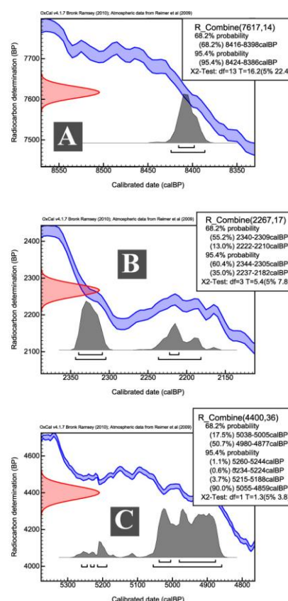
Figure IV.8 : Trois exemples d'applications du programme OxCal dont l'objectif est de déterminer un âge statistique pour des éruptions pour lesquelles on dispose de plusieurs datations radiocarbones. A : Ponomareva et al. (2004), B et C : Hidalgo et al. (2008). Rc (moyenne pondérée), Sc (déviation standard) et T (résultat du test du \chi^2 ) ont été directement calculé par OxCal. ΔRi et ΔSi caractérisent respectivement la variabilité des âges radiocarbones et de leurs erreurs analytiques.
