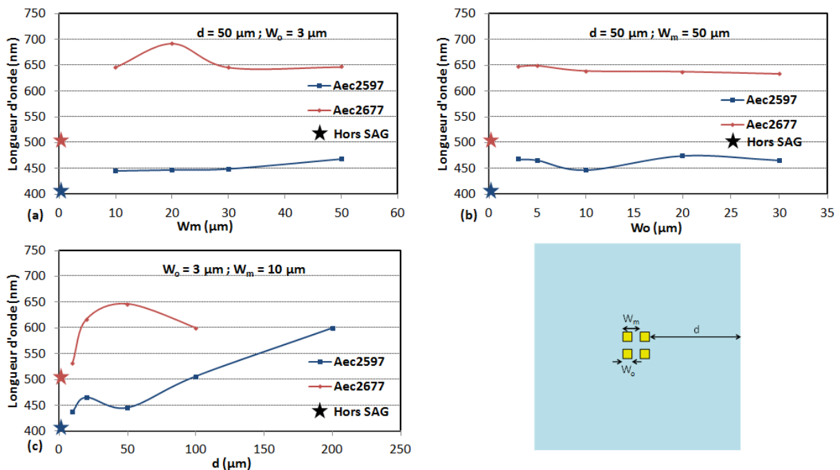
Figure 4-35 : Évolution de la longueur d'onde de structures MQW InGaN/GaN épitaxiées sélectivement à 805 °C en fonction des dimensions de motifs « 2x2 ». Les débits de TEGa sont respectivement de 16 et 24 sccm pour Aec2597 et Aec2677 (tableau 4-9). Le premier présente une sélectivité totale, tandis que des polycristaux se forment en surface du masque diélectrique pour des dimensions d \geq 80 \mu m .
