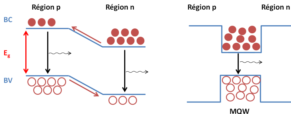
Figure 1-15 : Représentation d'une homojonction p - n (à gauche) et d'une hétérojonction p - n (à droite).
