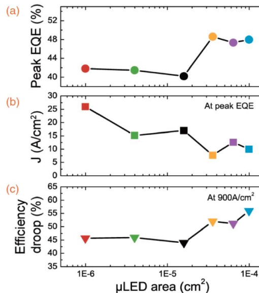
Figure 1-22 : Rendement maximal (a), densité de courant au rendement maximal (b), et chute d'efficacité à 900 A/cm 2 (c) en fonction de la taille des LEDs [54].
