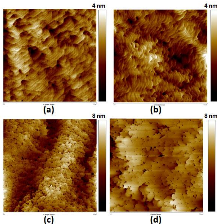
Figure 4-2 : Images AFM en champ 5x5 µm de « template » GaN sur substrat saphir (a et c) et d'une couche de GaN déposée sélectivement sur ces « templates » (b et d). La rugosité élevée d'un « template » se répercute sur la qualité de la couche déposée sélectivement.
