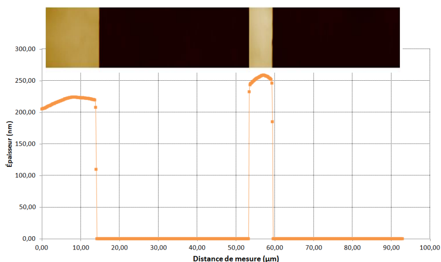
Figure 4-8 : Mesure AFM d'un motif « bandes » de largeur W_m = 40 \mu m et d'ouverture W_o = 5 \mu m d'une croissance SAG de GaN (échantillon Aec2579).
