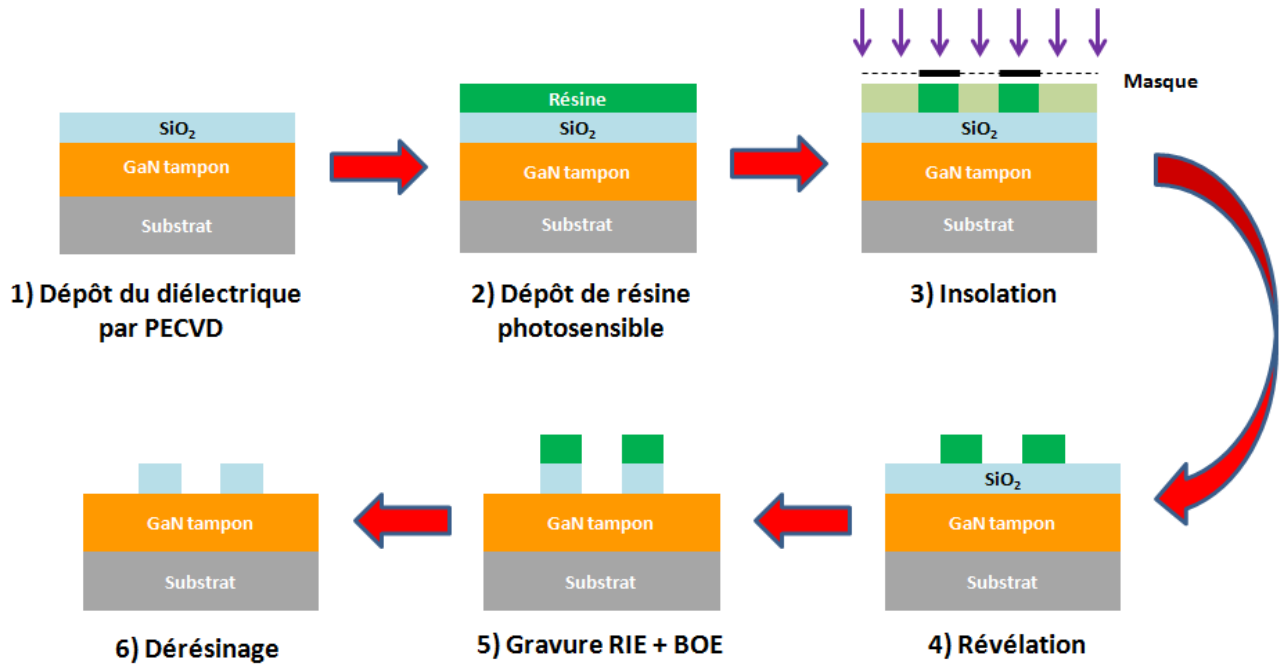
Figure 2-12 : Procédé de photolithographie de fabrication des « templates ».
