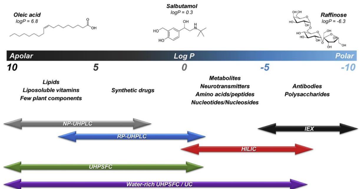
Figure 10 : Gamme de polarité des composés analysables selon la technique chromatographique, repris de [127]
