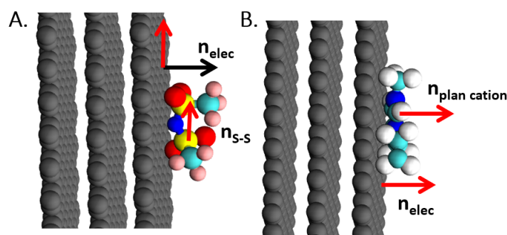
FIGURE 6.14 – Schéma explicatif pour le calcul des angles entre les ions du système [LiB]_{10} et l'électrode. (A) Pour le groupement TFSl, (B) pour le groupement BMIM.
