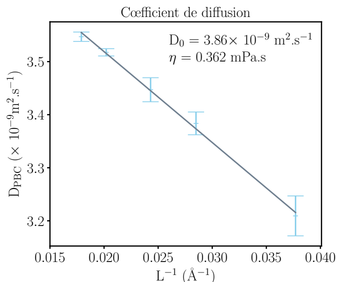
FIGURE 3.5 – Coefficient de diffusion de l'acétonitrile D_{\text{PBC}} pour cinq boîtes de simulations, en fonction de l'inverse de la taille de la boîte L . Les barres d'erreurs correspondent à l'intervalle de confiance à 95 %.[94]
