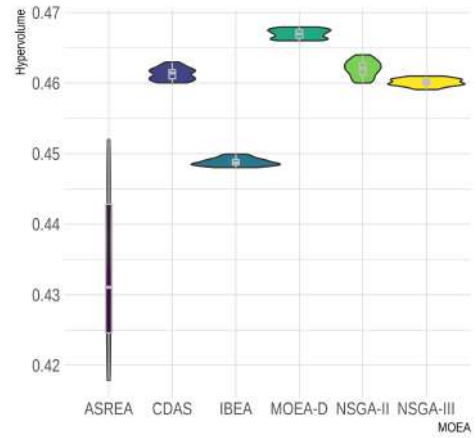
b) DTLZ2
