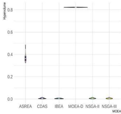
a) DTLZ1
