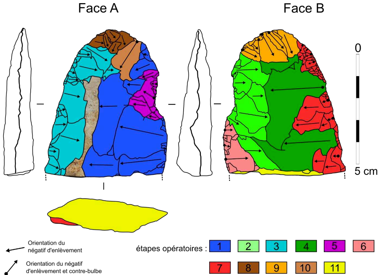
Figure 262. Pont-de-Planches – Fragment de pièces foliacée biface, répartition des étapes opératoires, des contre-bulbes et direction des négatifs d'enlèvements (DAO : T. Desmadryl).
