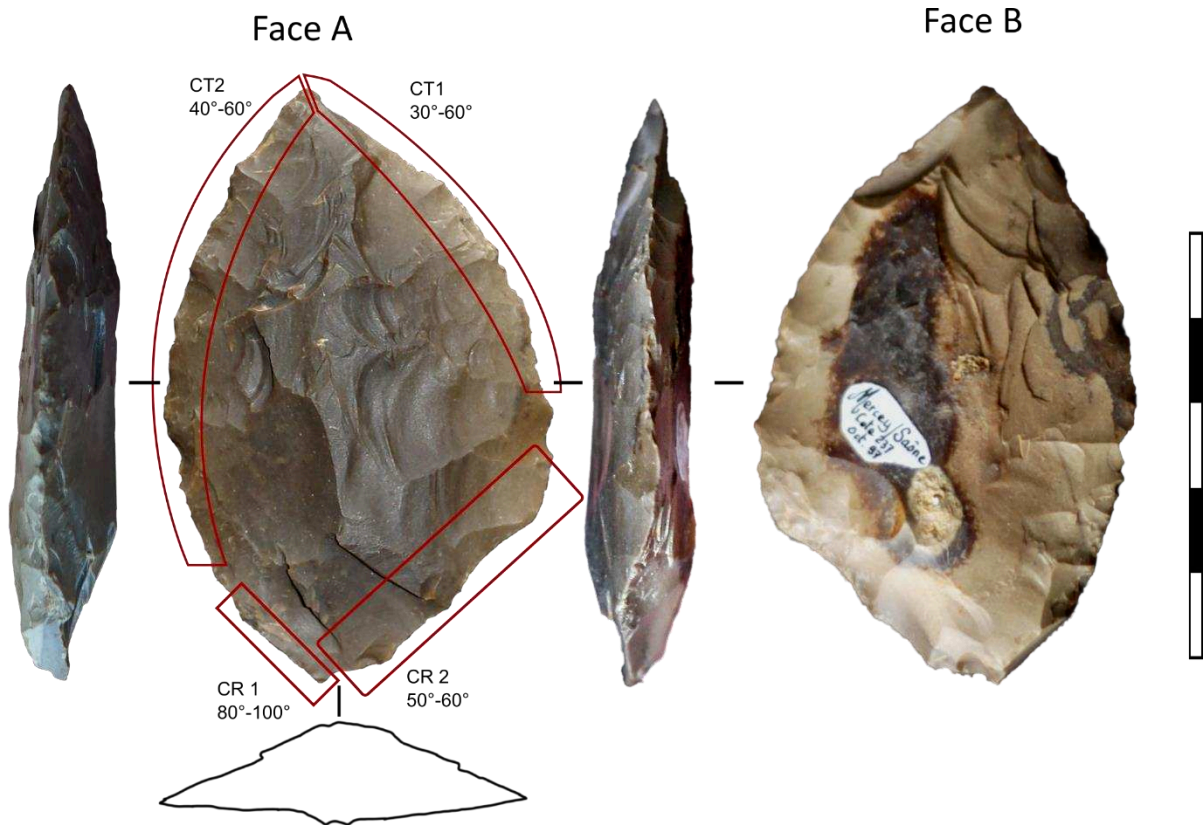
Figure 186. Mercey-sur-Saône – Localisation des unités techno-fonctionnelles de contact transformatif ou réceptif (Photos et D.A.O. : T. Desmadril).
