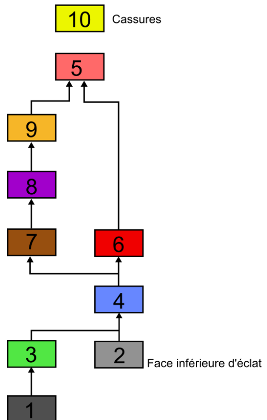
Figure 220. Velleuxon « Champ du Pâlis » - Diagramme représentant la succession en chronologie relative des étapes opératoires de façonnage de la pointe foliacée bifaciale (DAO : T. Desmadryl).
