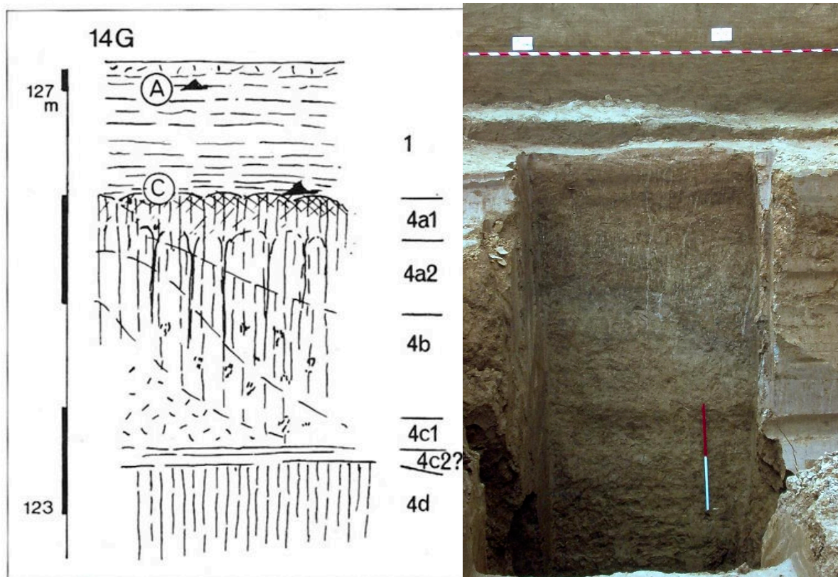
Figure 60. Rencourt-lès-Bapaume – Chantier Nord, coupe 14G. 1 : limons brun jaunâtre à litage épais ; 4a 1 : sol gris forestier ; 4a 2 : B(t)g de sol brun lessivé avec traces d'hydromorphie et gélifluxion ; 4b : limon argileux brun à tâche d'hydromorphie ; 4c1 : limon brun-jaune avec tâches d'hydromorphie ; 4c2 : limon brun jaune clair ; 4d : paléosol brun rouge (d'après Tuffreau, 1993, Photo : A. Tuffreau).
