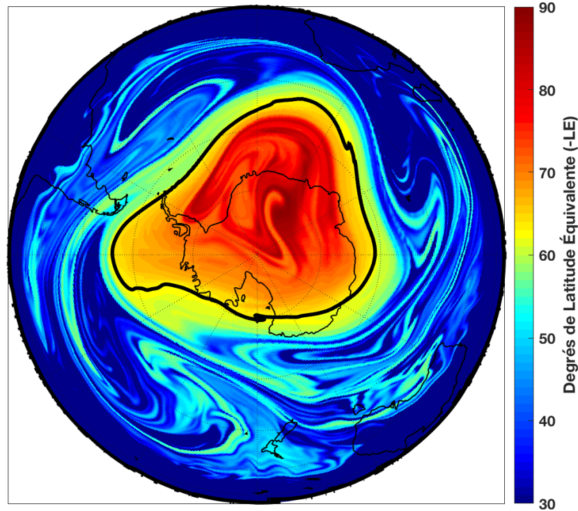
FIGURE 2.4 – Carte de latitude équivalente en °LE, au niveau isentrope 475 K le 15 octobre 2007 à 12UT dans l’hémisphère sud. Elle est obtenue à partir des sorties de simulation du modèle numérique MIMOSA à 3° x 3° de résolution spatiale. Comme pour la PV, la LE inversée (-LE) est représentée pour faciliter la représentation du vortex lorsque nous le représentons dans l’hémisphère sud, et elle le sera dans tout le reste du manuscrit pour cet hémisphère. Le champ de LE décrit fidèlement le champ de la PV. La valeur maximale de la LE (-/+90° selon l’hémisphère) représente ainsi la région du maximum de PV. L’intérieur du contour noir épais (50 PVU, environ 63,5°LE) représente l’intérieur du vortex (le vortex principal).
