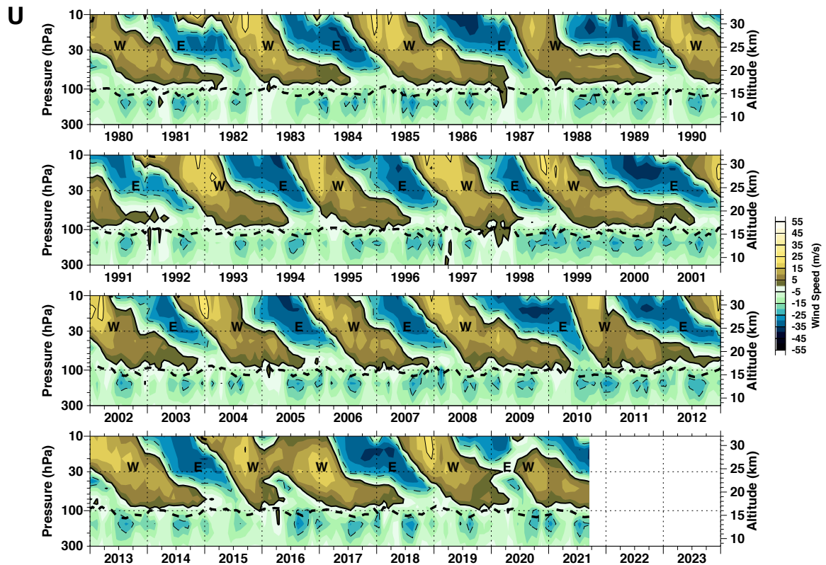
FIGURE 1.8 – Vent moyen mensuel zonal U ( \text{m}\cdot\text{s}^{-1} ) dérivé des radiosondes de Singapour ( 1^\circ\text{N} , 104^\circ\text{E} ) entre 10 et 300 hPa de 1980 à septembre 2021. Les différentes couleurs représentent un écart de 5\text{m}\cdot\text{s}^{-1} les unes des autres. Les zones en bleu/vert représentent un vent négatif (d’est) et les zones en marron/jaune représentent un vent positif (d’ouest). Les contours sont placés tous les 20\text{m}\cdot\text{s}^{-1} , avec des pointillés pour les vents d’est et des traits pleins pour les vents d’ouest, ainsi qu’un vent nul en noir plus épais. La ligne tiretée noire épaisse représente la tropopause. [Source : https://acd-ext.gsfc.nasa.gov/Data_services/met/qbo/qbo.html ].
