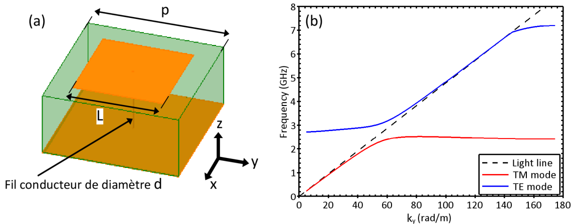
Figure 5.11: (a) Cellule élémentaire de la métasurface AMC à mushroom. (b) Diagramme de dispersion pour L = 13\text{ mm} et p = 18\text{ mm} .
