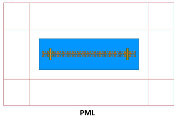
Figure 3.3: (a) Excitation de la ligne en méandre par des antennes dipôles. (b) Utilisation des conditions PML pour créer un modèle ouvert autour de la structure.
