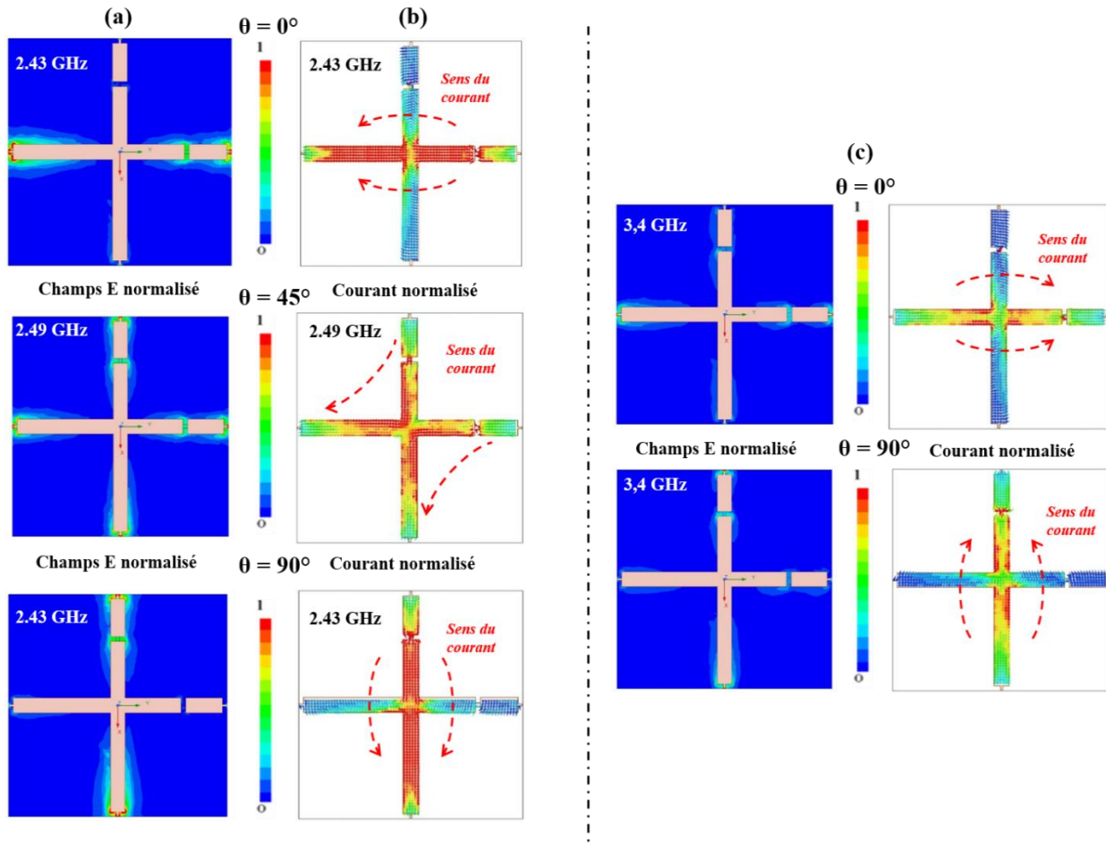
Figure 98: Cartographie de la structure DCK pour \varphi= 0^\circ, 45^\circ, \text{ et } 90^\circ , (a) Champs E normalisé à la fréquence d'absorption maximale. (b) Courant surfacique avec des flèches rouges indiquant le sens du courant. (c) Cartographie des champs pour le seconde pic d'absorption à 3.4 GHz.
