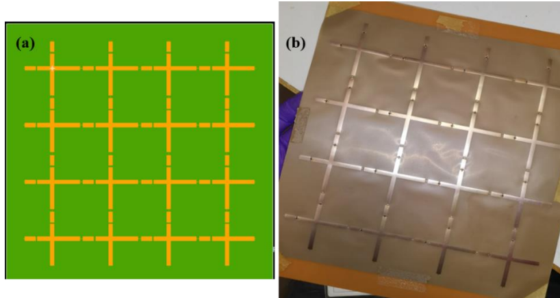
Figure 133: Image de la métasurface issue du fichier de fabrication Gerber (a), (b) Métasurface fabriquée comprenant 4×4 des dipôles croisés sur le substrat de Kapton de type II.
