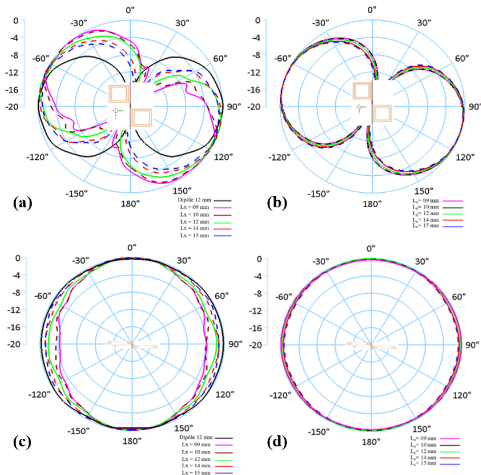
Figure 49: Diagramme de rayonnement de l'antenne à SRRs. Gain normalisé en dB pour L_x variable, à gauche pour la fréquence du 1er dip de réflexion et à droite pour la fréquence du second dip de réflexion. (a) et (b) : azimut, (c) et (d) : élévation.
