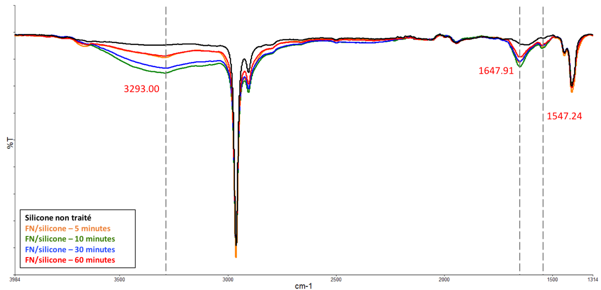
Figure 88: Spectres infrarouges des surfaces de silicone nues avant et après 5 (orange), 10 (vert), 30 (bleu), 60 minutes (rouge) d'adsorption de la fibronectine
