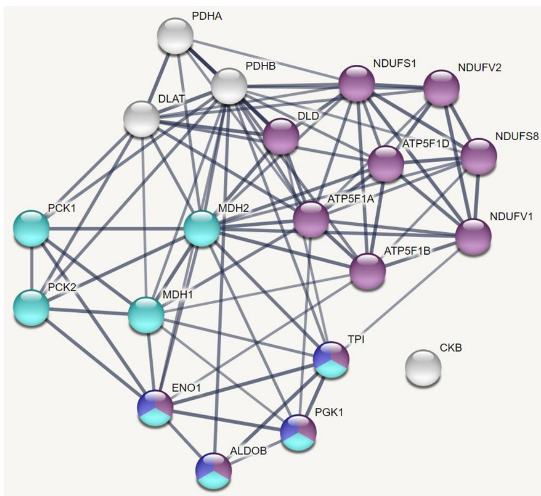
Figure 49 : String Interactions au sein de la catégorie METABOLISME ENERGETIQUE. En violet, protéines du processus biologique GO 0046034 ATP, processus métaboliques ; en bleu foncé, protéines du processus biologique GO 0061621, Glycolyse canonique ; en bleu turquoise, protéines du processus biologique GO 0006094, Néoglucogénèse. L'épaisseur des traits représente le niveau de confiance des interactions détectées par String ( https://string-db.org/Interactions ).
