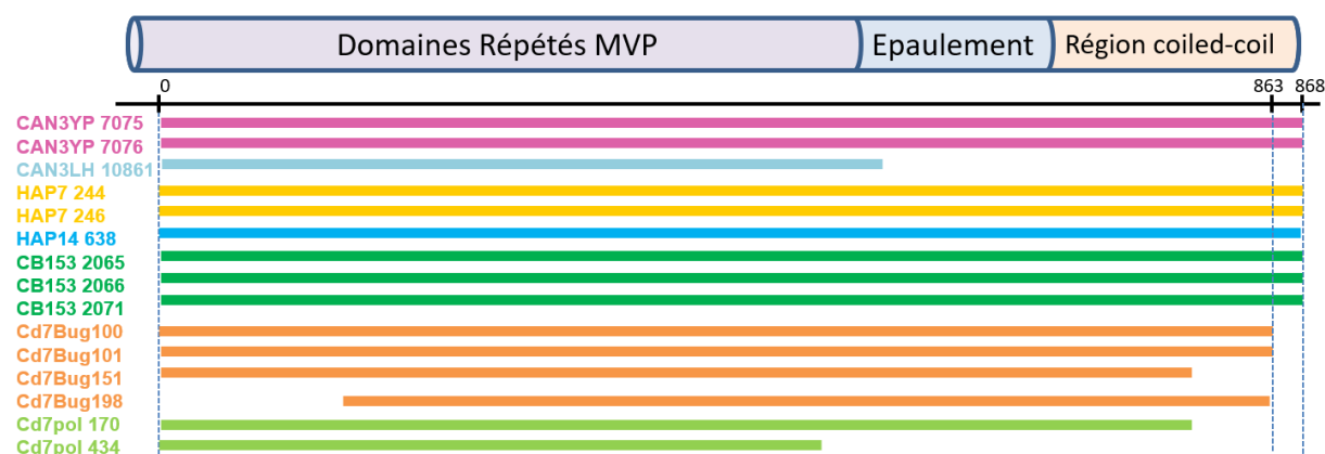
Figure 37 : Schématisation des zones de recouvrement de la MVP pour les protéoformes identifiées dans les différentes études. Chaque protéoforme est désignée par le code de l'étude dont elle est issue associé à son numéro de spot.
