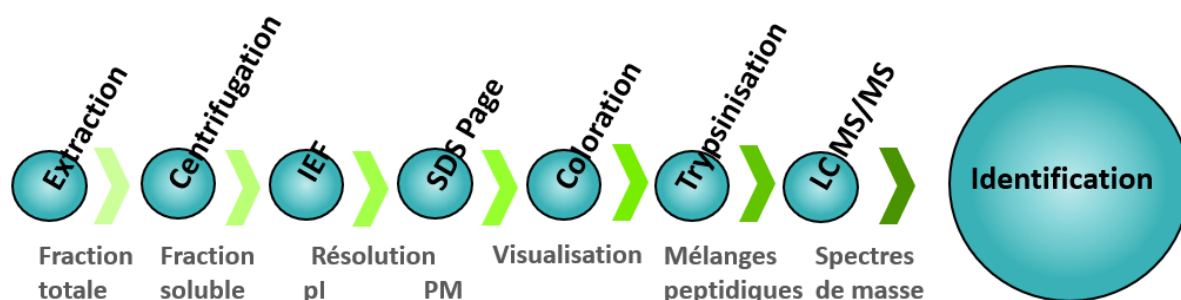
Figure 15 : Stratégie d'analyse protéomique par électrophorèse bidimensionnelle. Les protéines solubles sont obtenues après broyage dans un tampon d'extraction et centrifugation. Le mélange est séparé par isoélectrofocalisation (IEF) et électrophorèse dénaturante sur gel de polyacrylamide (SDS-PAGE). La séparation est visualisée par coloration au bleu colloïdal. Après analyse d'image, les protéoformes d'intérêt sont excisées des gels et digérées par trypsinisation. Les peptides résultants sont analysés par spectrométrie de masse après séparation par chromatographie liquide (LC MS/MS).
