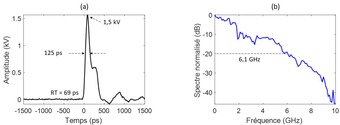
Figure III.23 : (a) Profil temporel de l'impulsion unipolaire g n r e par une ligne de 2 cm et (b) son profil spectral.
