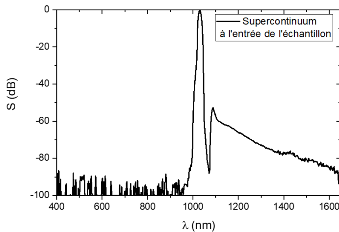
Figure II.40 : Spectre supercontinuum généré dans un cristal Nd 3+ :YAG filtré par un Notch 1064 nm et un LP1064 nm et envoyé sur l'échantillon pour réaliser des mesures M-CARS (3 ps, 41 mW, 4,1 μJ – 1.4 MW, 10 kHz).
