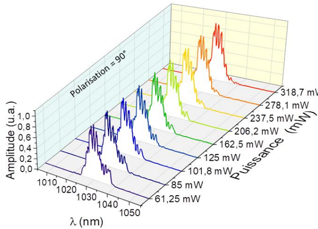
Figure II.22 : Exemple de l'évolution du spectre de l'onde pompe après sa propagation dans le PPLN ( T = 200^\circ\text{C} ) en fonction de la puissance moyenne pour une polarisation de 90^\circ ( \chi^{(3)} ) et une durée d'impulsion de 3 ps.
