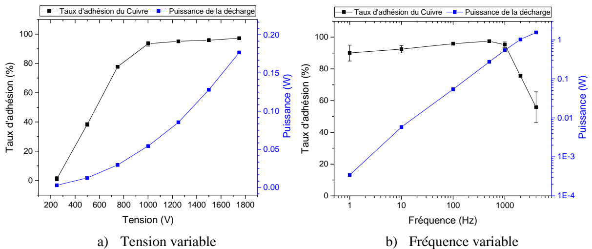
Figure V.36. Evolution de la récupération des particules de cuivre en fonction de la tension et de la fréquence pour le cas de l'actionneur correspondant au rapport g/w = 1 . Conditions : Tensions carrée ; E_r = 1000 V/mm ; f = 100 Hz.
