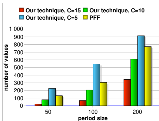
(d) CH_2, \mathcal{V} = 10
