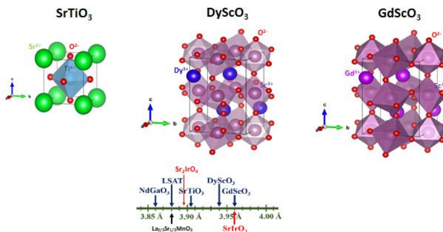
Figure 3.2 : Mailles élémentaires de \text{SrTiO}_3 (cubique), \text{DyScO}_3 (orthorhombique) et \text{GdScO}_3 (orthorhombique) ainsi qu'une comparaison de leur paramètre de maille pseudocubique notamment avec celui de \text{SrIrO}_3
