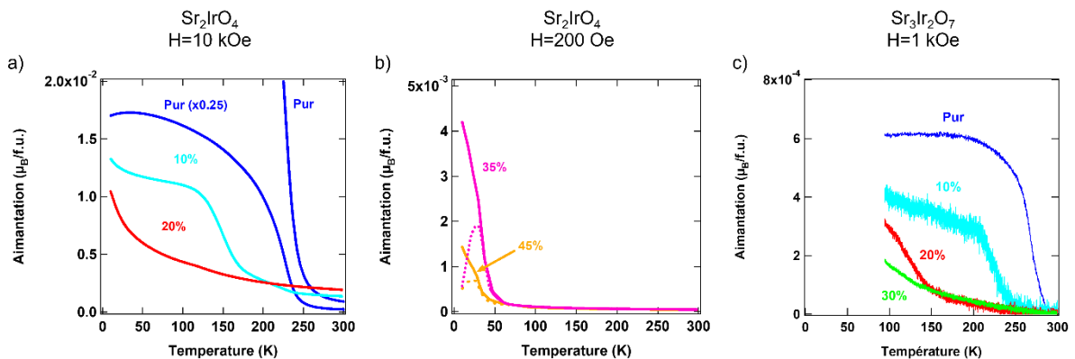
Figure 5.9 : Aimantation de monocristaux substitués en Ru de a) \text{Sr}_2\text{IrO}_4 (SQUID, H=10\text{ kOe} ), b) \text{Sr}_2\text{IrO}_4 (SQUID, H=200\text{ Oe} ) et de c) \text{Sr}_3\text{Ir}_2\text{O}_7 (VSM, H=1000\text{ Oe} ). Trait plein : refroidissement sous champ, pointillés : refroidissement en champ nul.
