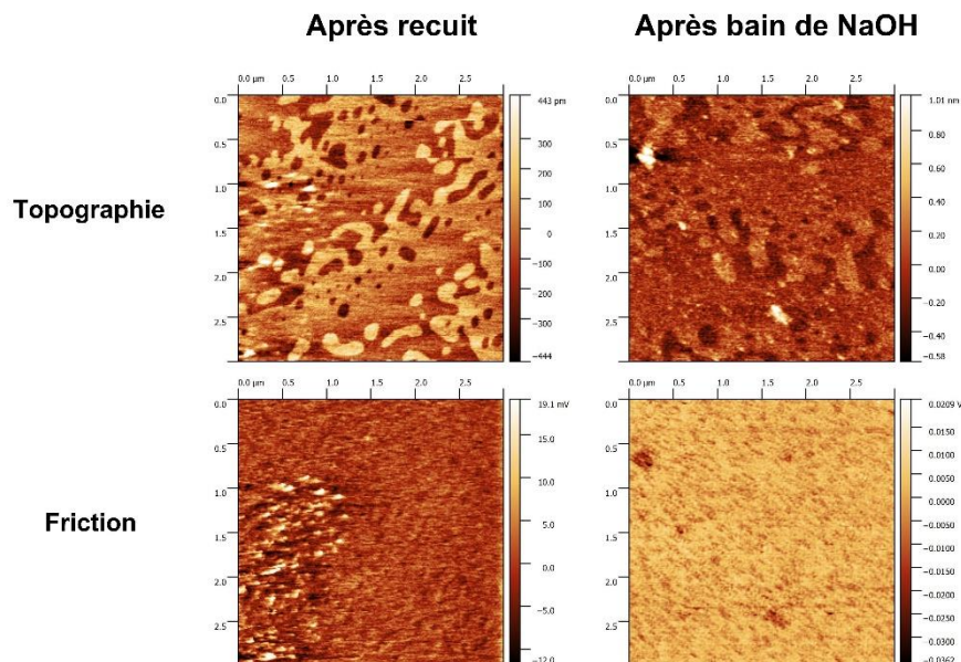
Figure 3.9 : Images AFM de topographie et de friction réalisées en mode contact sur un substrat de GdScO_3 (110) après le recuit à 1000\text{ }^\circ\text{C} et le bain dans une solution de NaOH .
