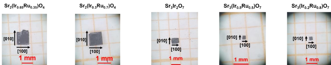
Figure 5.2: Images optiques de cristaux de Sr 2 IrO 4 et Sr 3 Ir 2 O 7 substitués au ruthénium.
