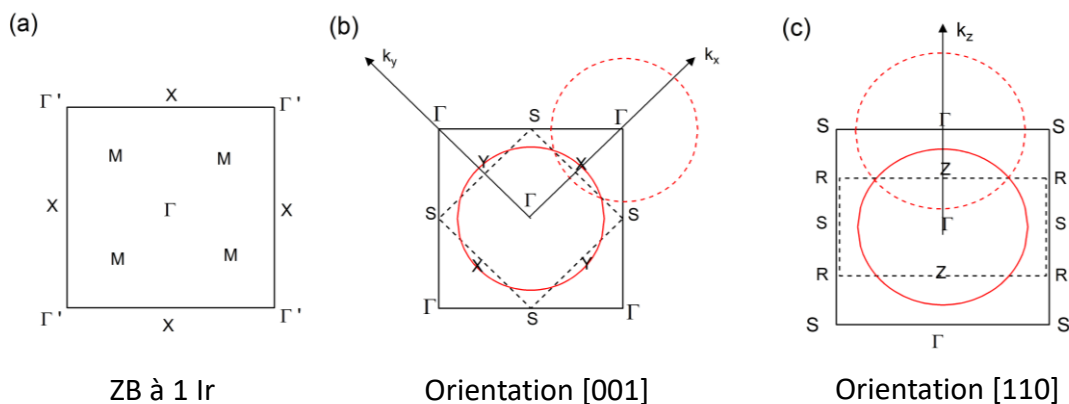
Figure 4.16 : Zones de Brillouin 2D et points de haute symétrie pour (a) une maille fictive pseudo-cubique (ZB à 1Ir), (b) le plan (001) de la ZB 3D de SrIrO 3 à k_{\text{perp}}=0 , (c) le plan (110) de cette maille à k_{\text{perp}}=0 . Le carré noir représente à chaque fois la ZB à 1Ir et le carré pointillé la coupe de la ZB 3D. Le cercle rouge symbolise une surface de Fermi isotrope et le cercle pointillé son repliement par rapport au bord de zone (par souci de clarté, un seul de ces repliements est dessiné).
