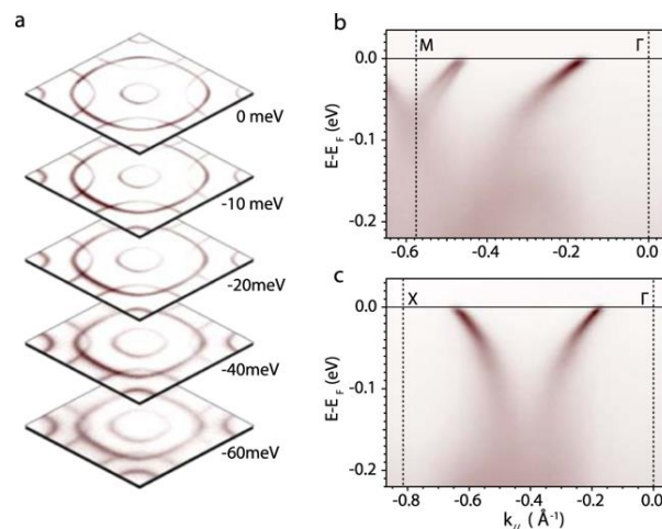
Figure 2.19 : Gauche : image isoénergétique d'ARPES. Droite images d'ARPES de \text{Sr}_2\text{RhO}_4 170
