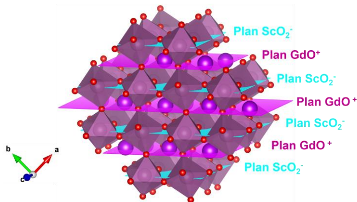
Figure 3.8 : Empilement des plans GdO^+ et ScO_2^- dans le substrat GdScO_3 pour une terminaison (110)
