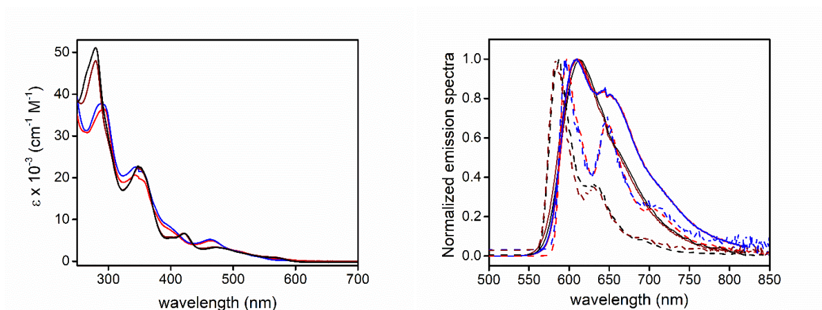
Figure 8. Spectres d'absorption électronique (à gauche) et d'émission (à droite) pour 4 (trace rouge), 5 (trace bleue), 6 (trace rouge foncé) et 7 (trace noire) dans le dichlorométhane à une concentration de 3,0 \times 10^{-5} M en condition dégazée (traces solides) et dans la matrice vitreuse 2-MeTHF à 77 K (traces pointillées). Les échantillons ont été excités à \lambda_{exc} = 420, 460 et 480 nm pour le composé 4,5,6 et 7 , respectivement.
